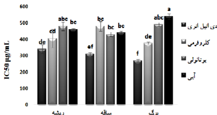
شکل ۲- مقایسه مقادیر IC 50 اجزای عصاره متانولی حاصل از اندام‌های مختلف (برگ، ساقه و ریشه) گیاه سدابی جنوبی بر رده سلولی سرطانی RAJI (حروف متفاوت نشان دهنده تفاوت معنی دار در سطح p ≤ 0.05 است).
