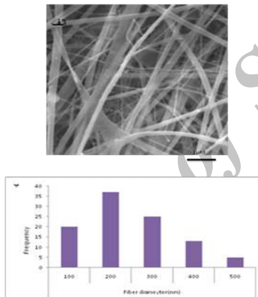
شکل ۱- میکروگراف میکروسکوپ الکترونی SEM. الف- نانوفیبرهای داربست الکترواسپینینگ PCL. ب- نمودار میانگین قطر فیبرهای داربست نانوالیاف PCL که میانگین بیش‌ترین الیاف حدوداً ۲۰۰ نانومتر اندازه‌گیری شد (scale bar: 1 \mu m).
