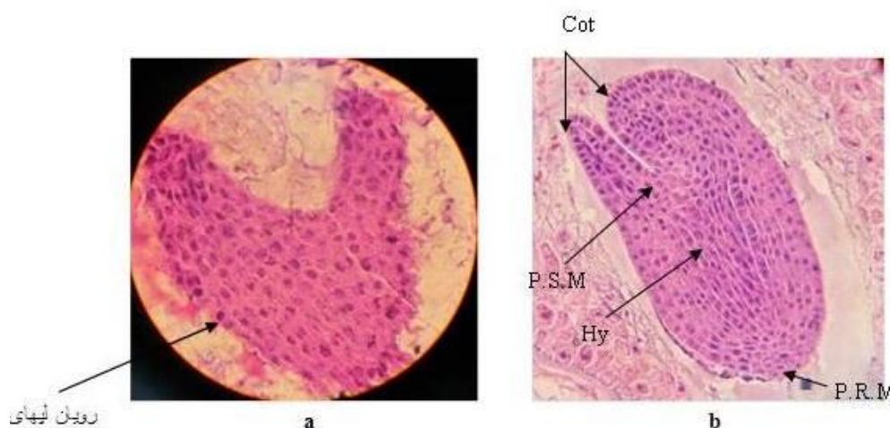
شکل ۱۶- برش طولی بذر (a: رویان لپه ای، b: رویان اژدری) (Cot: لپه، P.R.M: پرومریستم ریشه، P.S.M: پرومریستم ساقه، Hy: هیپوکوتیل). بزرگنمایی x ۱۹۲۰. Fig. 16. Longitudinal section of seed (a: Cotyledon embryo, b: Torpedo-shaped embryo) (Cot: Cotyledon, P.R.M: Root Pro-Meristem, P.S.M: Stem Pro-Meristem, Hy: Hypocotyle). Magnified by 1920x.
