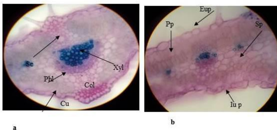
شکل ۵- برش عرضی برگ (a: رگبرگ اصلی، b: رگبرگ فرعی). (Col: کلانشیم، Sc: مجرای ترشچی، Phl: فلوم، Xyl: زایلوم، Cu: کوتیکول، Sp: پارانشیم اسفنجی، Pp: پارانشیم نردبانی). بزرگنمایی x ۷۶۸.
