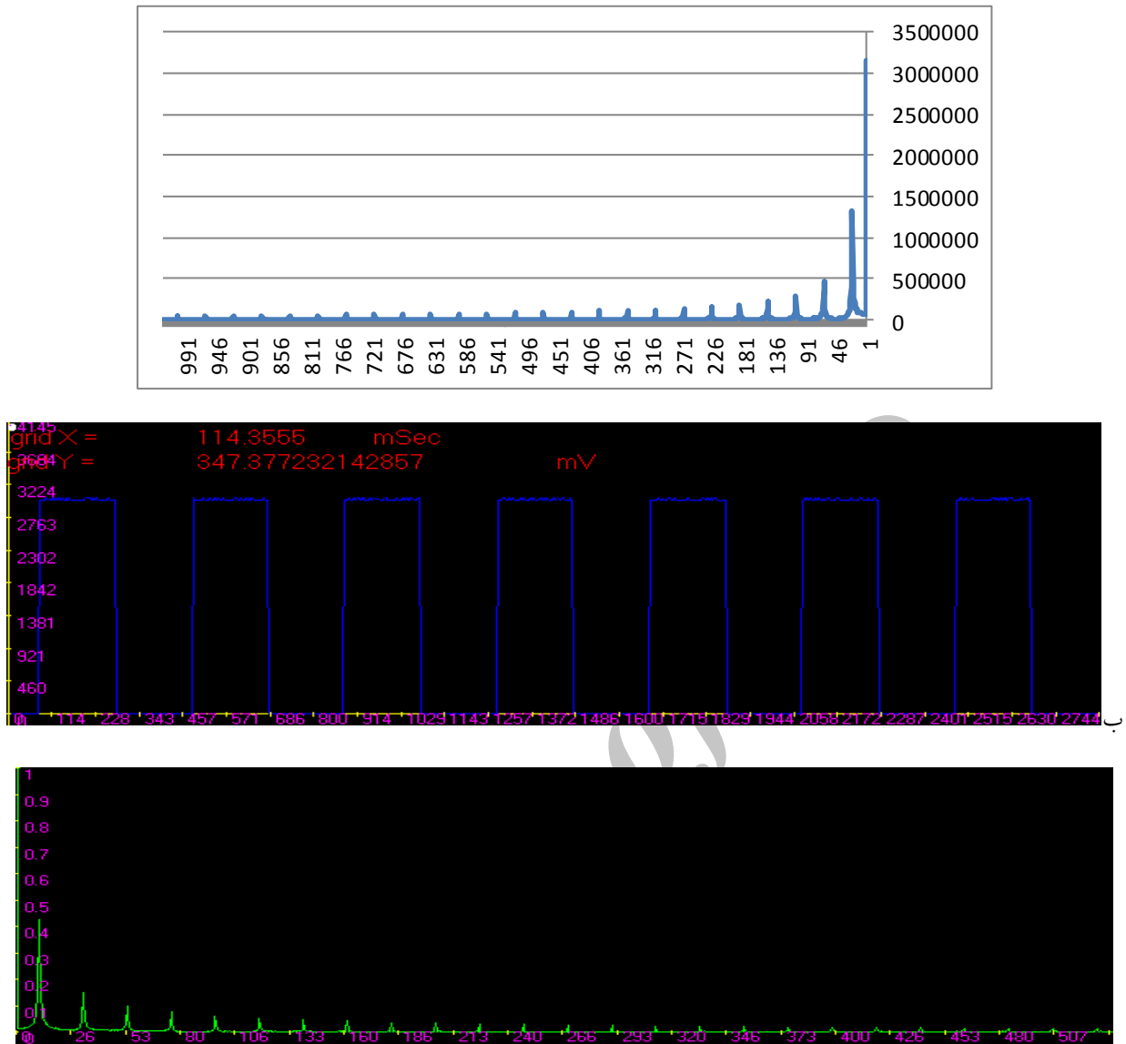
شکل ۴- نمودار طیف ولتاژ بر حسب زمان و دامنه ولتاژ حالت الف) بدون ماده، ب) با ماده.
