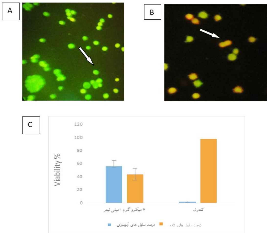
شکل ۳- رنگ آمیزی اکریدین اورنج / پروپیدیوم یدید. A در گروه کنترل، سلول‌ها به رنگ سبز مشاهده می‌شوند که نشان دهنده زنده بودن سلول‌ها است. B در نمونه‌های تیمار با غلظت ۴ میکروگرم بر میلی لیتر نانو ذره نقره، تعدادی از سلول‌ها به رنگ زرد و نارنجی مشاهده می‌شوند که نشان می‌دهند این سلول‌ها دچار آپوپتوز شده‌اند. C : نمودار نشان می‌دهد که درصد زیست پذیری سلول‌ها تحت تیمار با غلظت ۴ میکروگرم / میلی لیتر نانو ذرات نقره کاهش یافته است (بزرگنمایی × ۲۰۰).
