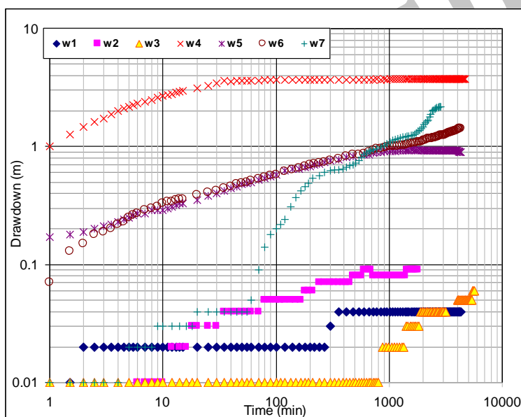
شکل ۵. نمودارهای افت-زمان مربوط به آزمایش پمپاژ چاه های آهکی منطقه مورد مطالعه
