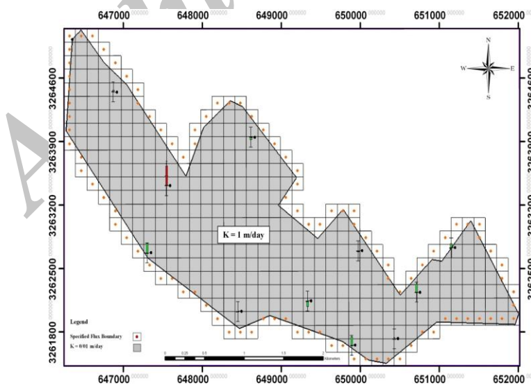
شکل ۲. شبکه تفاضلات محدود و مقدار هدایت هیدرولیکی واسنجی شده برای آیخوان شهرک صنعتی بزرگ شیراز
