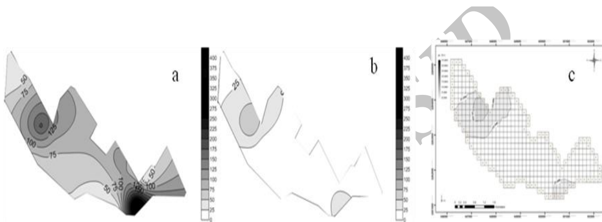
شکل ۵- a. غلظت اولیه نیکل در آبان ۱۳۸۶. b. غلظت مشاهده ای نیکل در بهمن ۱۳۸۶. c. غلظت محاسبه شده نیکل توسط مدل در بهمن ۱۳۸۶
