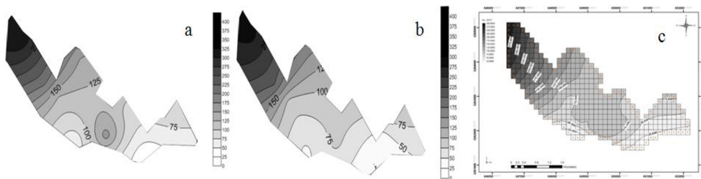
شکل ۸- a. غلظت اولیه مولیبدن در شهریور ۱۳۸۶. b. غلظت مشاهده ای مولیبدن در اردیبهشت ۱۳۸۷. c. غلظت محاسبه شده مس توسط مدل در اردیبهشت ۱۳۸۷
