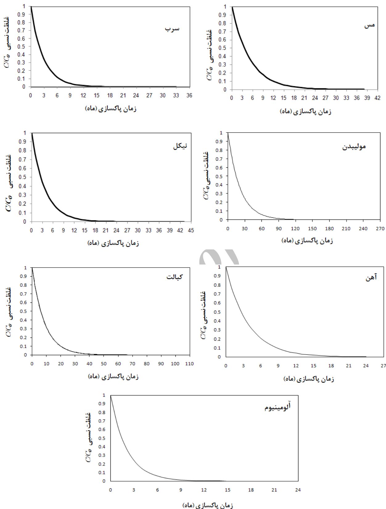
شکل ۱۲. نمودار تغییرات غلظت نسبی عناصر Al و Fe, Ni, Cu, Pb, Mo, Co نسبت به زمان
