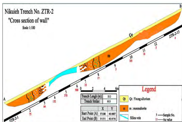
شکل ۲. ترانشه حفر شده روی رگه اصلی (دید به سمت شمال) که در طرح شماتیک آن موقعیت دگرسانی های گرمایی ایجاد شده در اطراف رگه نشان داده شده است.
