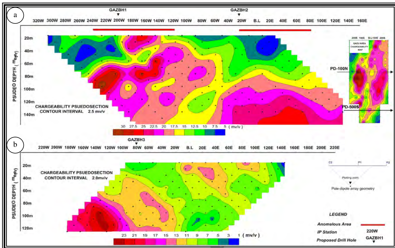
شکل ۱۱. (a) شبه مقطع ۱۰۰N. (b) شبه مقطع ۵۰۰S. (شرکت مهندسی مشاور کان ایران، ۱۳۸۵)
