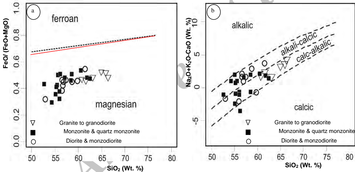
شکل ۸. (a) نمودار FeO/(FeO+MgO) در مقابل SiO_2 . مرز آهن و منیزیم (خط چین، Frost et al. 2001) با تغییراتی (خط ممتد) توسط Frost and Frost, (2008) استفاده از FeO/(FeO+MgO) = 0.46 + 0.005SiO_2 که در آن FeO = FeO + 0.9Fe_2O_3 نشان داده شده است. توده‌های نفوذی منطقه مورد مطالعه در محدوده منیزیم قرار می‌گیرد. (b) موقعیت توده‌های نفوذی بر روی نمودار Na_2O+K_2O-CaO در مقابل SiO_2 .
