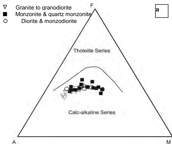
شکل ۶. (a) نمودار AFM جهت تفکیک سنگ‌های آذرین کالک آلکان از تولیتی (Irvine & Baragar, 1971) و (b) نسبت \text{K}_2\text{O} به \text{SiO}_2 در توده‌های نفوذی منطقه (Peccerillo & Taylor, 1976)
