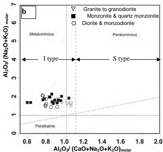
شکل ۵. نمودار طبقه‌بندی سنگ‌های آذرین درونی بر اساس مجموع \text{Na}_2\text{O} و \text{K}_2\text{O} در مقابل \text{SiO}_2 (Middlemost, 1994). (b) نمودار نسبت \text{Al}_2\text{O}_3/(\text{Na}_2\text{O} + \text{K}_2\text{O}) در مقابل \text{Al}_2\text{O}_3/(\text{CaO} + \text{K}_2\text{O} + \text{Na}_2\text{O}) (Maniar and Piccoli, 1989). خط A/CNK=1.1 محدوده I ( A/CNK < 1.1 ) و S ( A/CNK > 1.1 ) را از یکدیگر جدا می‌کند (Chappell and White, 2001).
