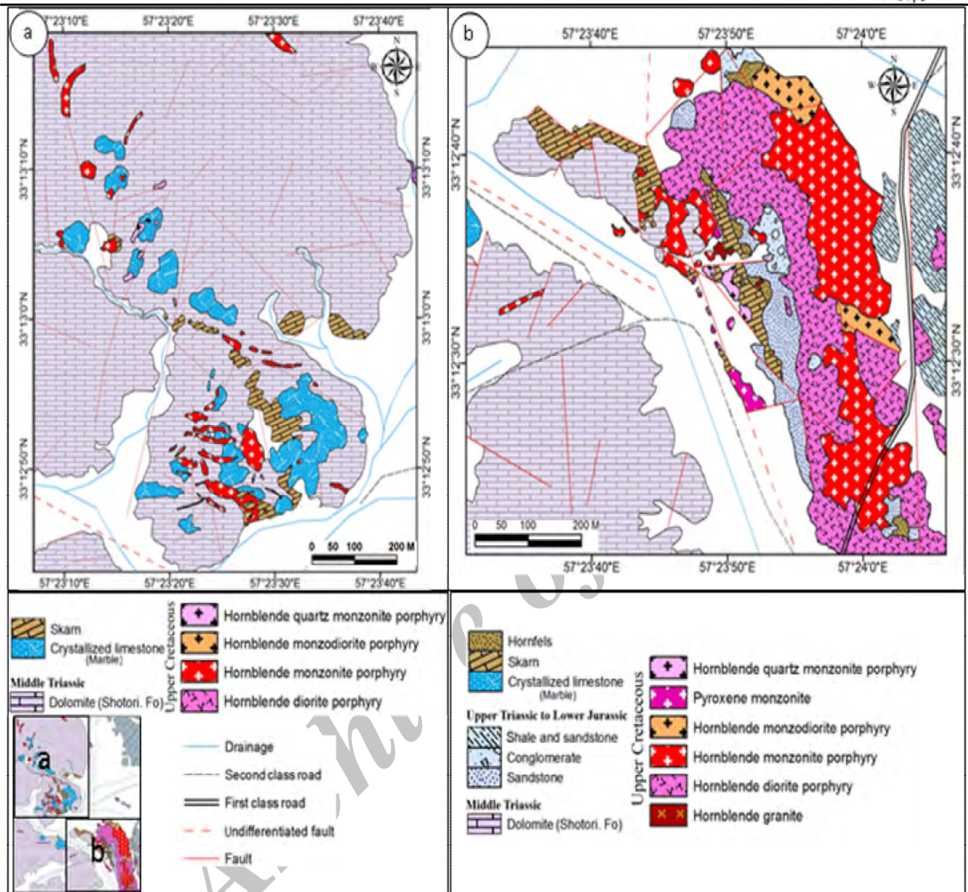
شکل ۴. نقشه زمین شناسی ۱:۱۰۰۰ منطقه کانه دار (a) بخش شمال غرب GA.I و (b) بخش جنوب شرق GA.I. اثرات دگرگونی همبری در امتداد نفوذ توده های نیمه عمیق بین دولومیت سازند شتری و شیل و ماسه سنگ شمشک قابل مشاهده است.
