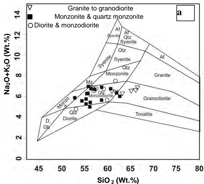
شکل ۵. نمودار طبقه‌بندی سنگ‌های آذرین درونی بر اساس مجموع \text{Na}_2\text{O} و \text{K}_2\text{O} در مقابل \text{SiO}_2 (Middlemost, 1994). (b) نمودار نسبت \text{Al}_2\text{O}_3/(\text{Na}_2\text{O} + \text{K}_2\text{O}) در مقابل \text{Al}_2\text{O}_3/(\text{CaO} + \text{K}_2\text{O} + \text{Na}_2\text{O}) (Maniar and Piccoli, 1989). خط A/CNK=1.1 محدوده I ( A/CNK < 1.1 ) و S ( A/CNK > 1.1 ) را از یکدیگر جدا می‌کند (Chappell and White, 2001).
