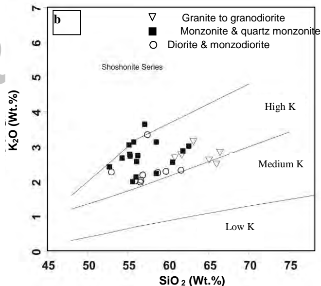
شکل ۶. (a) نمودار AFM جهت تفکیک سنگ‌های آذرین کالک آلکان از تولیتی (Irvine & Baragar, 1971) و (b) نسبت \text{K}_2\text{O} به \text{SiO}_2 در توده‌های نفوذی منطقه (Peccerillo & Taylor, 1976)
