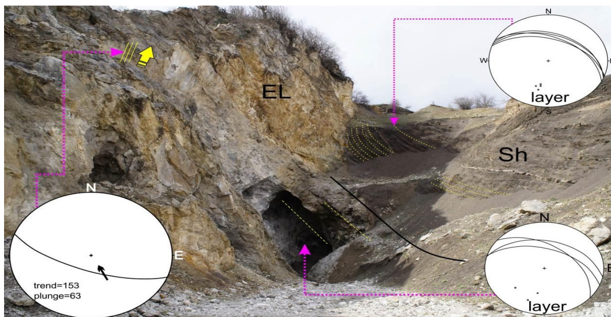
شکل ۱۳. نمایی از گسلش معکوس و صفحه گسل دروازه سنگ. تحت تاثیر این گسل، خمیدگی واحدهای شیلی (Sh) در مرز بین واحدهای آهکی-دولومیتی الیکا (El) دیده می شود، جهت دید به سمت شمال باختری.
