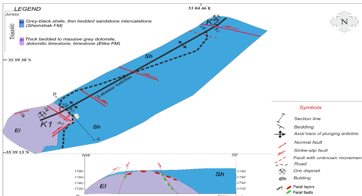
شکل ۳. نقشه زمین شناسی محدوده معدنی کمرپشت و مقطع ساختاری ترسیم شده در راستای مشخص شده. K1 محدوده معدنی کمرپشت-۱ و K2 محدوده معدنی کمرپشت-۲
