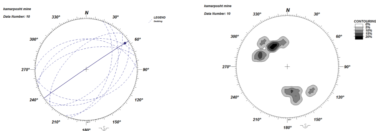
شکل ۶. نمودار کنتوری لایه بندی برداشت شده از طاقدیس لامرد معدن کمرپشت (تصویر سمت راست)، استریونت لایه بندی طاقدیس لامرد و موقعیت سطح محوری و محور طاقدیس لامرد (تصویر سمت چپ).
