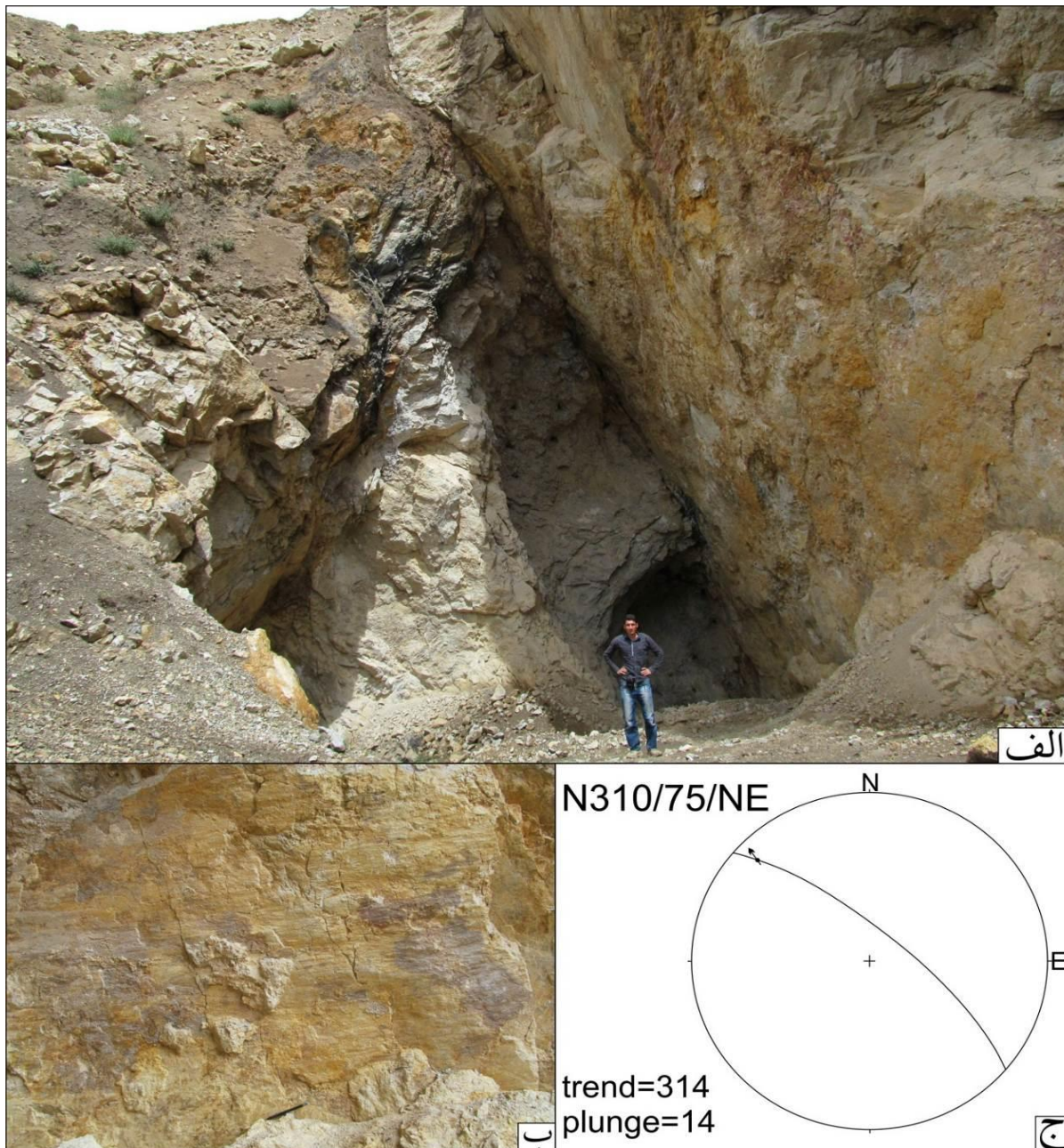
شکل ۱۲. الف: نمایی از گسل چپگرد لرزنه سر. در فرودبوار این گسل کانه‌زایی فلوریت دیده می‌شود. جهت دید شمال باختر. ب- پله‌های گسلی گسل لرزنه سر. ج- استریوگرام گسل چپگرد لرزنه سر.
