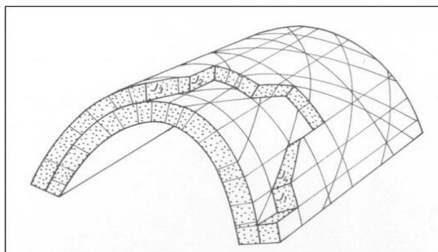
شکل ۱۵. نمایی شماتیک از شکستگی‌های ایجاد شده در حین چین خوردگی، شکستگی‌های دسته J1 از نوع عرضی و کششی، شکستگی دسته J2 از نوع طولی یا امتدادی و کششی، شکستگی‌های J3 و J4 از نوع مورب دارای مکانیسم امتدادلفز.
