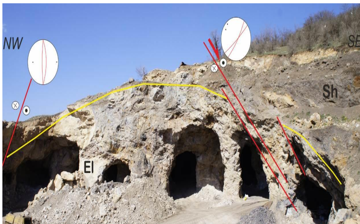
شکل ۴. نمایی از بخش مرکزی و تونل‌های حفاری معدن کمرپشت-۱، تونل‌ها به موازات محور طاقدیس حفاری شده است.
