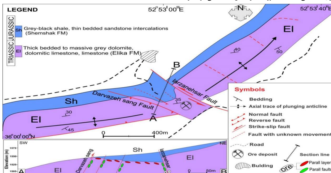
شکل ۹. نقشه زمین شناسی محدوده معدنی شش رودبار و مقطع ساختاری ترسیم شده در راستای مشخص شده.
