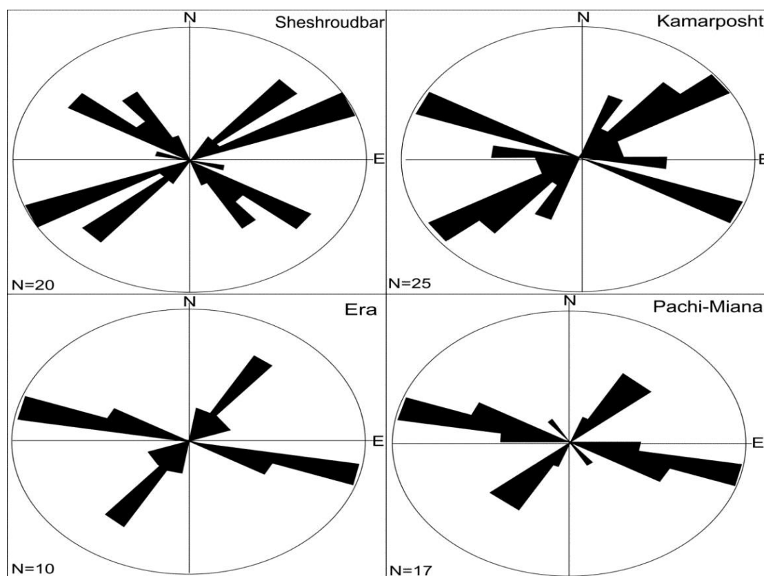
شکل ۱۶. نمودار گل سرخی امتدادی گسل‌ها و زون‌های گسلی فلئوریت دار معادن کمرپشت، شش رودبار، پاچی میانا و ارا.
