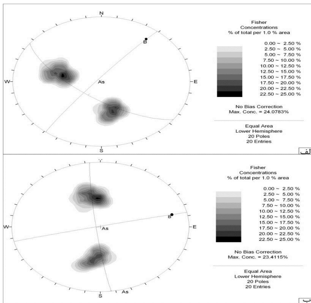
شکل ۱۰ الف. استریوگرام بخش شمال خاوری طاقدیس پالند رودبار. ب- استریوگرام بخش جنوب باختری طاقدیس پالند رودبار.
