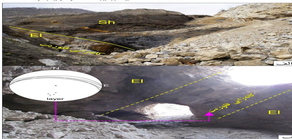
شکل ۱۴. الف) نمایی از واحدهای آهکی-دولومیتی الیکا (EI) با واحدهای شیلی-ماسه سنگی شمشک (Sh) در بین گسل های لرزه سر و دروازه سنگ. جهت دید شمال باختری. ب- نمایی از کانه زایی فلوریت در داخل تونل های حفاری شده. در این منطقه کانه زایی در واحد الیکا موازی با لایه بندی دیده می شود، جهت دید به جنوب جنوب خاوری.
