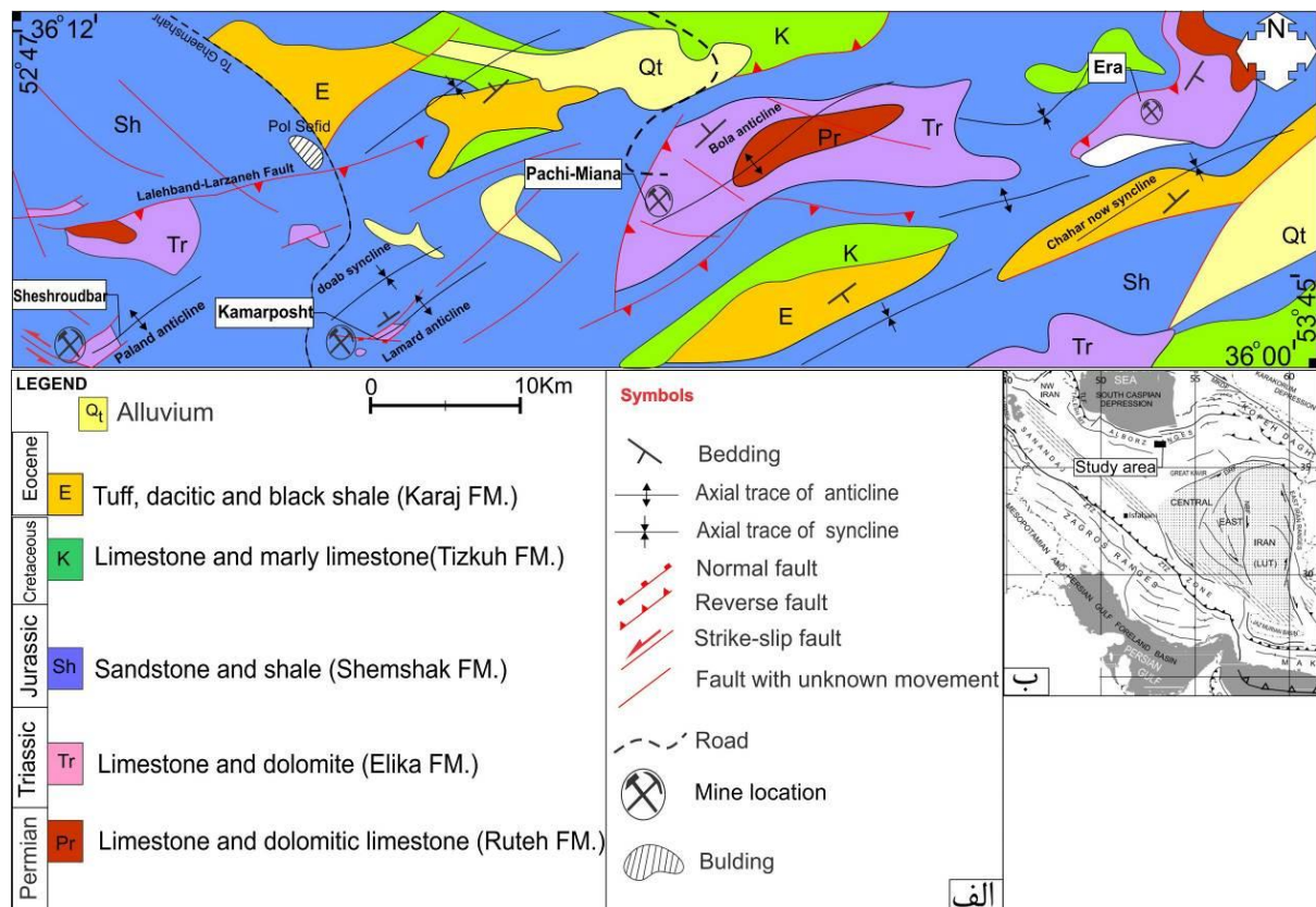
شکل ۱. الف) نقشه زمین شناسی ساده شده از نقشه ۱/۱۰۰۰۰۰ قائم شهر، کیاسر (سعیدی و اکبرپور، ۱۳۷۱)، پل سفید و نقشه سمنان با مقیاس ۱/۲۵۰۰۰۰ (Samadian et al., 1994) و موقعیت معادن فلوریت در مناطق سوادکوه، ختیرکوه و کیاسر (اصلاح شده از نبی‌لو و همکاران، ۱۳۹۲). ب) موقعیت منطقه مورد مطالعه (بر گرفته و ساده شده از Berberian and King, 1981)
