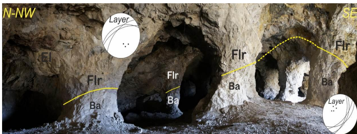
شکل ۵. نمایی از داخل تونل‌های بخش مرکزی معدن کمرپشت ۱- و موقعیت فلوریت چینه سان در واحد الیکا.
