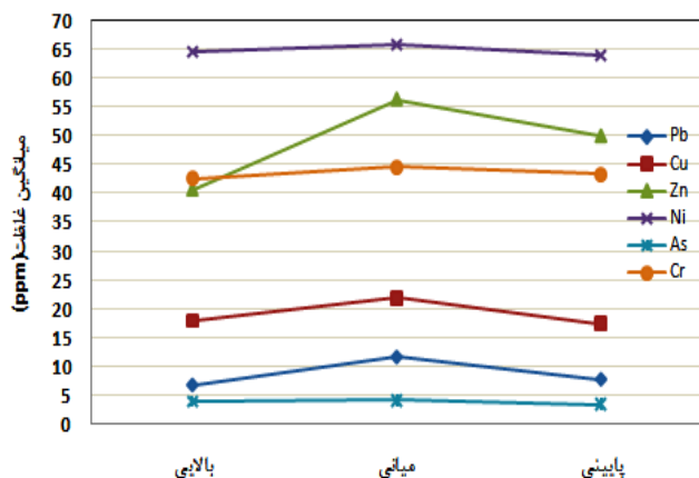
شکل ۳. میانگین غلظت فلزات در بخش های پایینی (ایستگاههای ۱-۸)، میانی (ایستگاههای ۹-۱۶) و بالایی (ایستگاههای ۱۷-۲۴) رودخانه کارون
