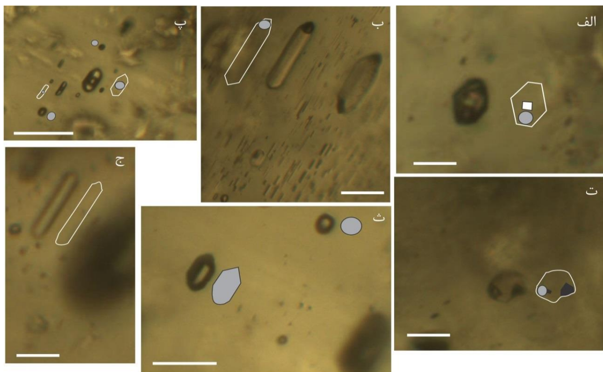
شکل ۸. تصاویری از انواع سیالات درگیر در آپاتیت. الف) نوع LVH، ب) نوع LV همراه با سیالات درگیر ثانویه عمدتاً از نوع L، پ) نوع LV همراه با V، ت) نوع LVO، ث) نوع V، و ج) نوع L. خط مقیاس برابر با ۱۰ میکرون است.
