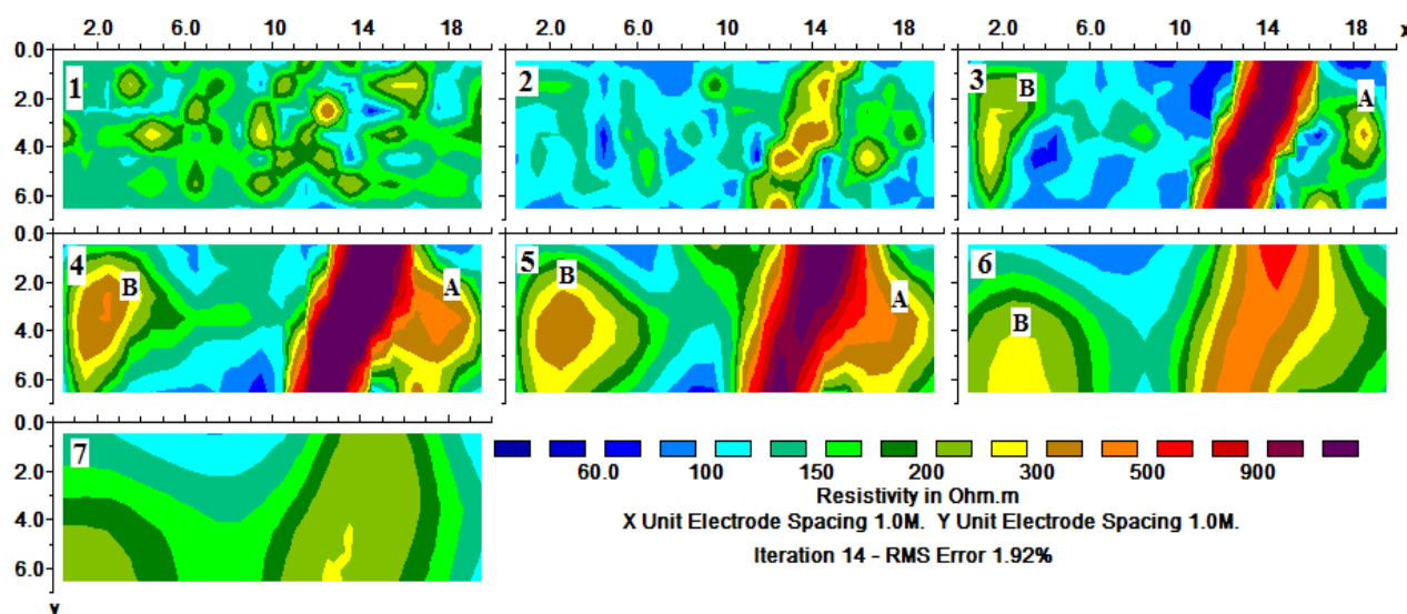
شکل ۸. لایه های افقی با ضخامت یک متر که توسط داده های مقاومت ویژه الکتریکی حقیقی بوسیله آرایه PD تهیه شده اند. عمق متناظر با لایه های این شکل عبارت است از: (۱) ۰/۵ - ۰ - ۱/۵ (۲)، ۰/۵ - ۲/۵ (۳)، ۱/۵ - ۳/۵ (۴)، ۲/۵ - ۳/۵ (۴)، ۳/۵ - ۴/۵ (۵)، ۴/۵ - ۷/۰ (۶)، ۴/۵ - ۷/۰ (۶)، ۷/۰ - ۹/۰ (۷) متر.
