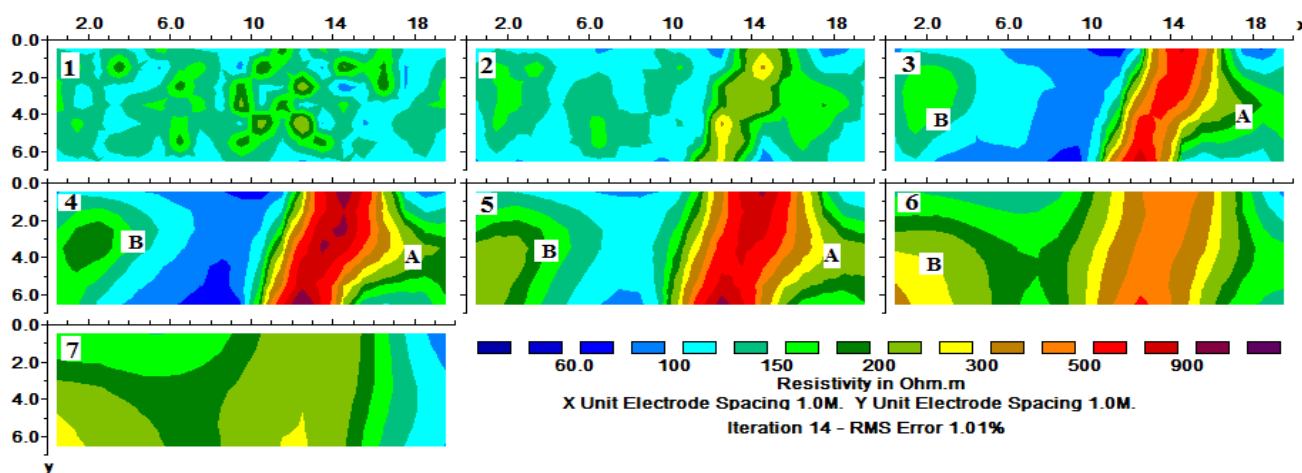
شکل ۹. لایه های افقی با ضخامت یک متر که توسط داده های مقاومت ویژه الکتریکی حقیقی بوسیله آرایه PP تهیه شده اند. عمق متناظر با لایه های این شکل عبارت است از: (۱) ۰/۵ - ۰ - ۱/۵ (۲)، ۰/۵ - ۲/۵ (۳)، ۱/۵ - ۳/۵ (۴)، ۲/۵ - ۳/۵ (۴)، ۳/۵ - ۴/۵ (۵)، ۴/۵ - ۷/۰ (۶)، ۴/۵ - ۷/۰ (۶)، ۷/۰ - ۹/۰ (۷) متر.
