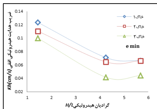
شکل ۹. ضریب نفوذپذیری افقی نمونه های غیر یکنواخت براساس گرادیان هیدرولیکی در شرایط حداقل تخلخل
