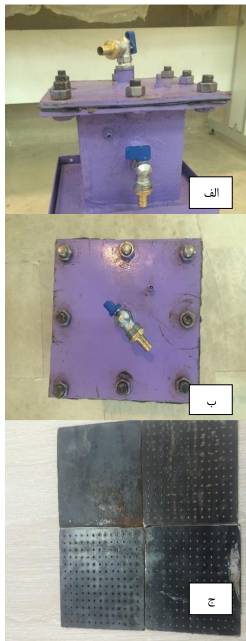
شکل ۴. نمایی از دستگاه نفوذپذیری افقی و عمودی و صفحات متخلخل
