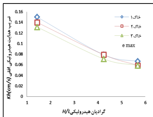
شکل ۱۰. ضریب نفوذپذیری افقی نمونه های غیر یکنواخت براساس گرادیان هیدرولیکی در شرایط حداکثر تخلخل
