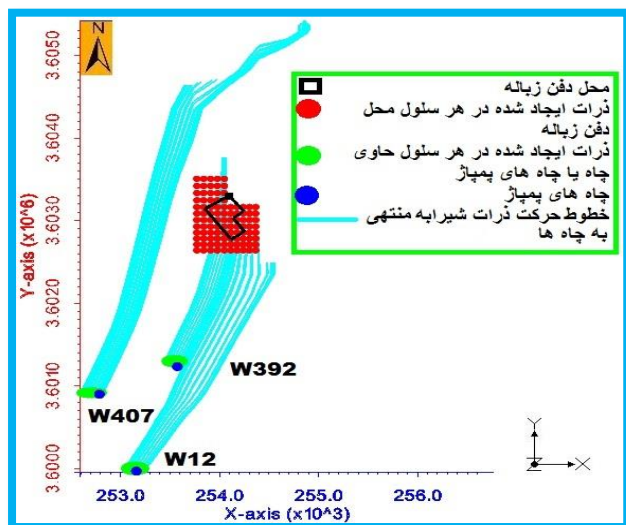
شکل ۲۰. شبیه سازی حرکت ذرات شیرابه منتهی به ۳ نمونه چاه پمپاژ موجود در آبخوان به روش پسر و با اعمال ۱۰ درصد کاهش پمپاژ.
