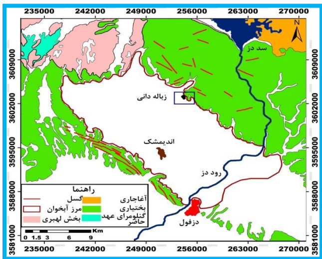
شکل ۱. نقشه زمین شناسی محدوده‌ی مورد مطالعه.
