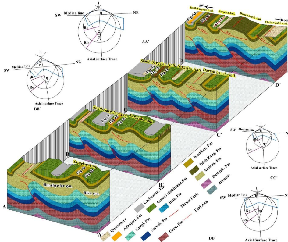
شکل ۳. بلوک دیاگرام نیمرخ‌های عرضی ساختاری در منطقه مورد مطالعه که محل این نیمرخ‌ها در (شکل ۱) مشخص شده است. شکل نحوه محاسبه پارامترهای هندسی و محل تصاویر صحرایی در هر نیمرخ نشان داده شده است.
