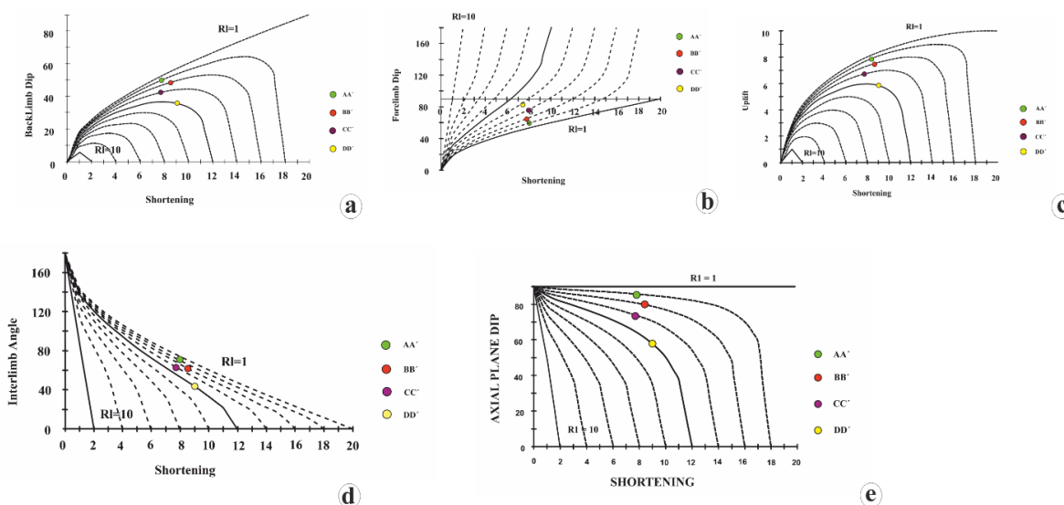
شکل ۸. نمودارهای تعیین پارامترهای هندسی چین‌های جدایشی (Poblet and McClay, 1996) منحنی‌های نمودارها، منطبق بر مقادیر RI به ترتیب ۱، ۱، ۱۱، ۱، ۲۵، ۱، ۴۳، ۱، ۶۷، ۲، ۲، ۵۰، ۳، ۳۳ و ۱۰ هستند (موقعیت تاقدیس سرگلان براساس پارامترهای هندسی آن بر روی نمودار نشان داده شده است).
