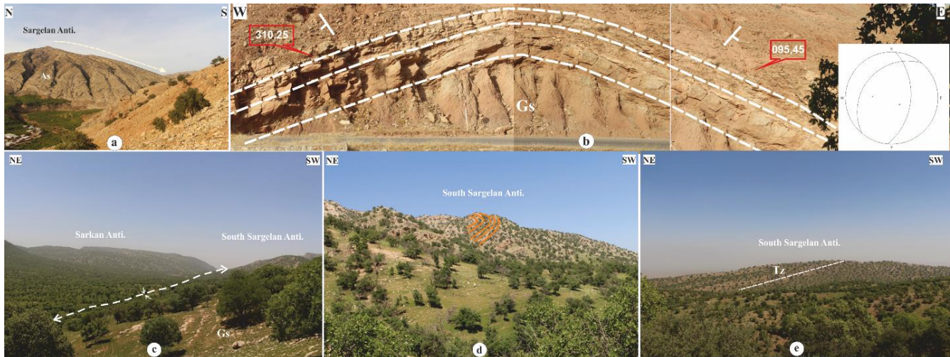
شکل ۴. (a) پلانژ تاقدیس سرگلان در امتداد نیمرخ ساختاری AA' با رخنمون سازند آسماری. (b) تاقدیس سطحی تشکیل شده در سازند گچساران در امتداد نیمرخ ساختاری AA' به علت عملکرد سطح جدایش بالایی به همراه تصویر استریوگرام. (c) محور ناودیس بین دو تاقدیس سرکان و سرگلان جنوبی با رخنمون سازند آسماری و گچساران در امتداد نیمرخ BB'. (d) یال جنوبی و برگشته تاقدیس سطحی سرگلان جنوبی با رخنمون سازند آسماری در امتداد نیمرخ BB'. (e) یال شمالی تاقدیس سرگلان جنوبی با رخنمون سازند آهکی آسماری و تله‌زنگ در امتداد نیمرخ BB'.
