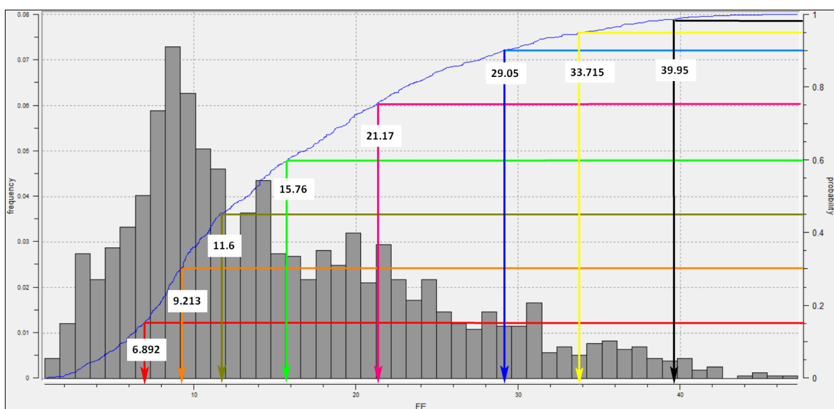
شکل ۹- تقسیم تابع توزیع تجمعی زون جنوبی کانسار چاه باشه به ۹ قسمت به منظور استفاده از کریجینگ شاخص متوالی.
