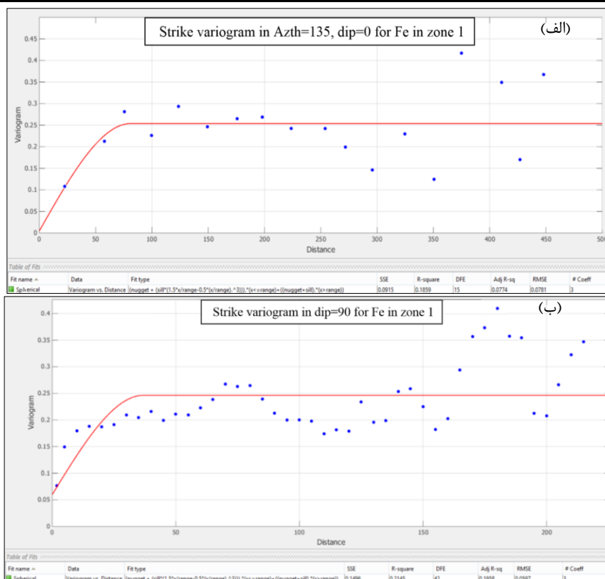
شکل ۶- واریوگرام های جهتی الف) آزیموت ۱۳۵ (شیب صفر درجه) و ب) شیب ۹۰ درجه برای داده های آهن زون ۱ در کانسار چاه باشه.
