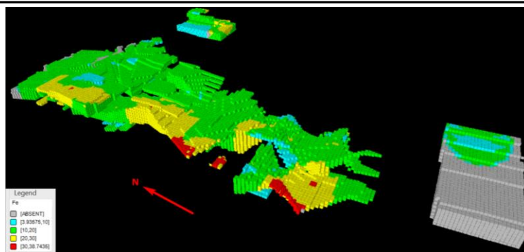
شکل ۸- نحوه توزیع عیار آهن در داخل مدل بلوکی زون جنوبی کانسار چاه باشه با روش عکس مجذور فاصله.
