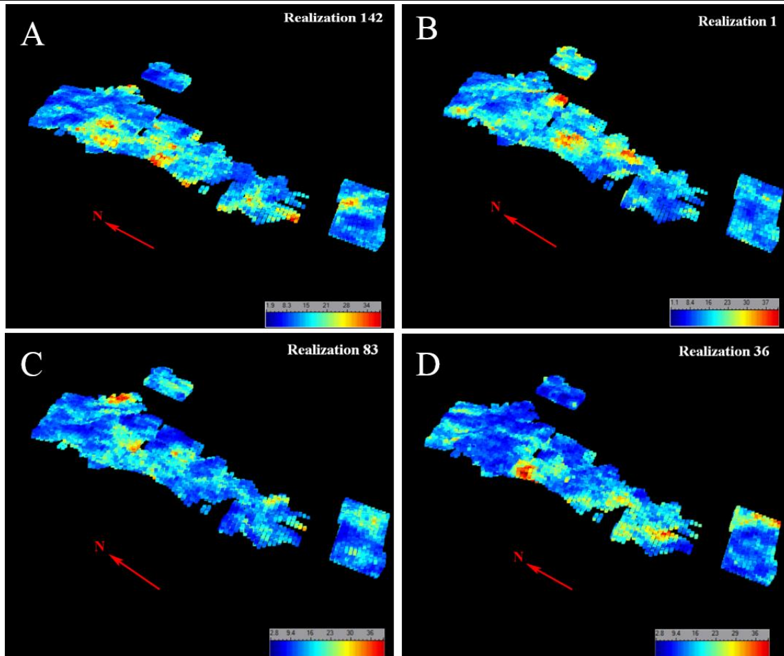
شکل ۱۴- نحوه توزیع عیار آهن مدل بلوکی برای چهار تحقق برتر. (A) تحقق شماره ۱۴۲، (B) تحقق شماره ۸۳، (C) تحقق شماره ۳۶، (D) تحقق شماره ۳۶.
