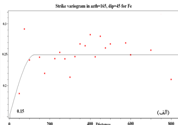
شکل ۱۰- واریوگرام های جهتی الف) آزیموت ۱۶۵ درجه و شیب ۴۵ درجه، ب) آزیموت ۱۰۵ درجه و شیب ۴۵ درجه جهت عملیات کریجینگ شاخص برای داده‌های آهن زون ۱ در کانسار چاه باشه.
