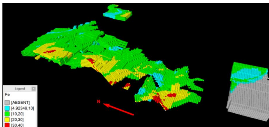
شکل ۷- نحوه توزیع عیار آهن در داخل مدل بلوکی زون جنوبی کانسار چاه باشه به روش کریجینگ معمولی.
