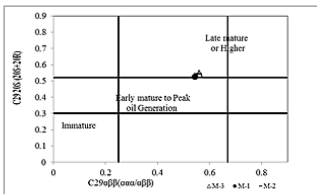
شکل ۵: نمودار نسبت C29\text{ Sterane } \alpha\beta/(\alpha\beta+\alpha\gamma) در برابر نسبت C29\text{ Sterane } 20S/(20S+20R) برای تشخیص میزان بلوغ نمونه مورد مطالعه (اقتباس از [۸]).
