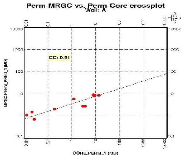
شکل ۵. نمودار متقاطع لاگ تراوایی تخمین زده شده به روش MRGC در مقابل تراوایی مغزه در چاه A.
