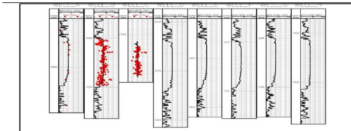
شکل ۷. تراوایی تخمین زده شده در چاه های مورد مطالعه به روش MRGC دواير قرمز رنگ مربوط به نتایج تراوایی آزمایشگاهی است.
