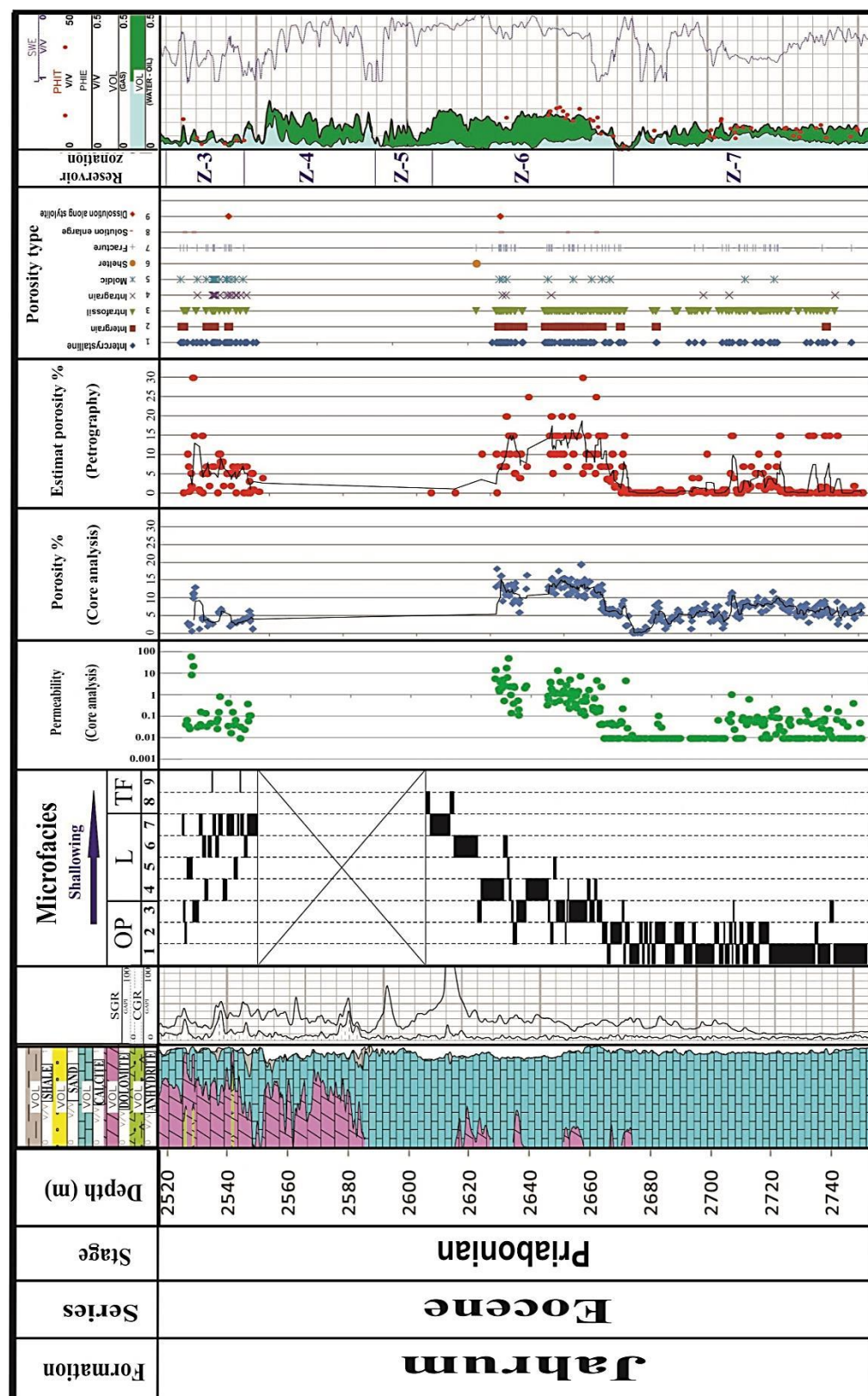
شکل ۳۱- انطباق داده‌های پتروگرافی با داده‌های پتروفیزیکی و مقایسه‌ی تخلخل حاصل از تخمین چشمی با تخلخل حاصل از آنالیز مغزه (سلیمی و همکاران، ۲۰۱۳) در سازند جهرم، میدان نفتی گلخاری (برگرفته از نقشه‌ی سازند آسماری و جهرم چاه شماره ۱۱ میدان نفتی گلخاری، شرکت ملی مناطق نفتخیز جنوب، اداره مهندسی پتروفیزیک).
