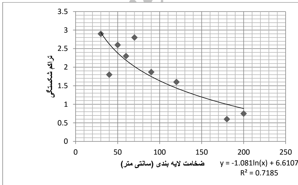
شکل ۱۱) نمودار نقطه‌ای بین تراکم شکستگی و ضخامت لایه بندی در سازند آسماری تاقدیس دارا.
