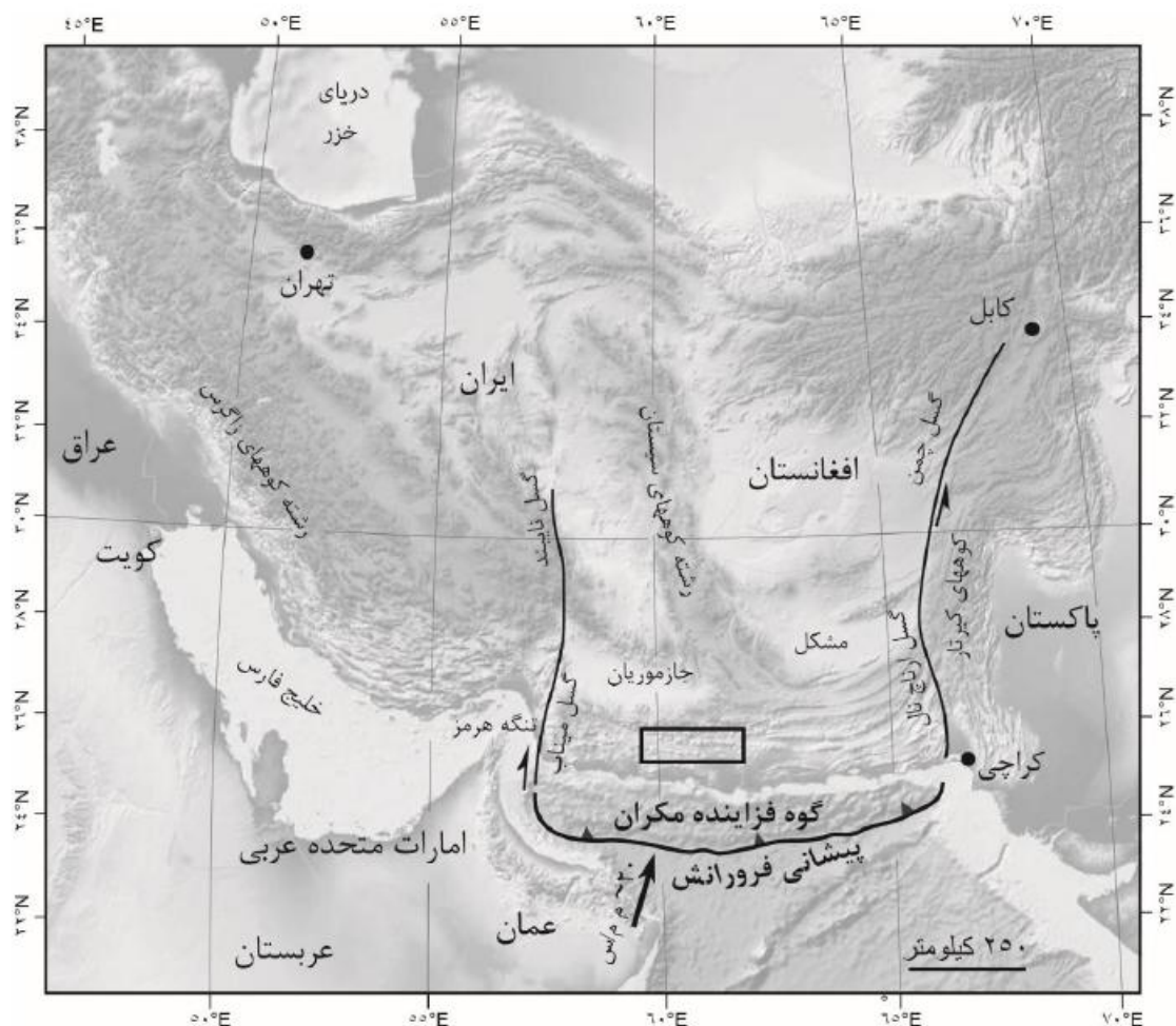
شکل ۱. موقعیت کلی زمین ساختی پائنه فزاینده مکران روی تصویر ETOP1 مستطیل کشیده شده موقعیت تقریبی شکل ۲ را به نمایش گذارده است. منبع تصویر پس زمینه http://www.ngdc.noaa.gov/mgg/global/relief/ETOP1
