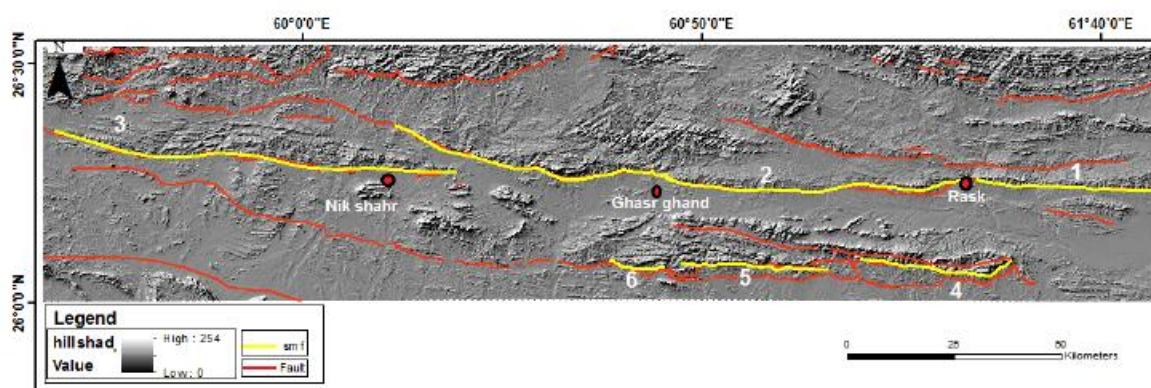
شکل ۴. شاخص پیشانی کوهستان در شش قسمت در گسل‌های قصرقند (۱ و ۲)، کهورکان (۳) و گنجان (۴، ۵ و ۶) محاسبه شده است. نتایج، فعالیت بالای زمین ساختی را نشان می‌دهد. تصویر زمینه مربوط به داده‌های رقومی با دقت ۱۰ متر، به صورت هیل‌شید، است.
