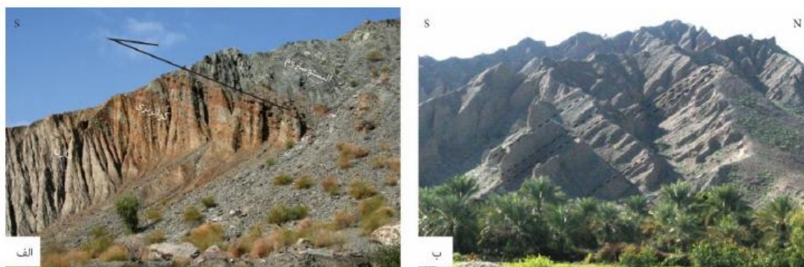
شکل ۳. (الف) نمایی از گسل قصرقند که باعث رانده شدن رسوبات ایستوستروم در بالا روی کنگلومرای کواترنری (رخنمون قهوه‌ای) و مارن (خاکستری روشن) شده است. (ب) نمایی کلی از کنگلومرای پلیوسن پلیستوسن در جنوب راسک (محل رخنمون در شکل ۲). خط چین سیاه رنگ روی تصویر جهت گیری لایه بندی عمومی را نشان می‌دهد.
