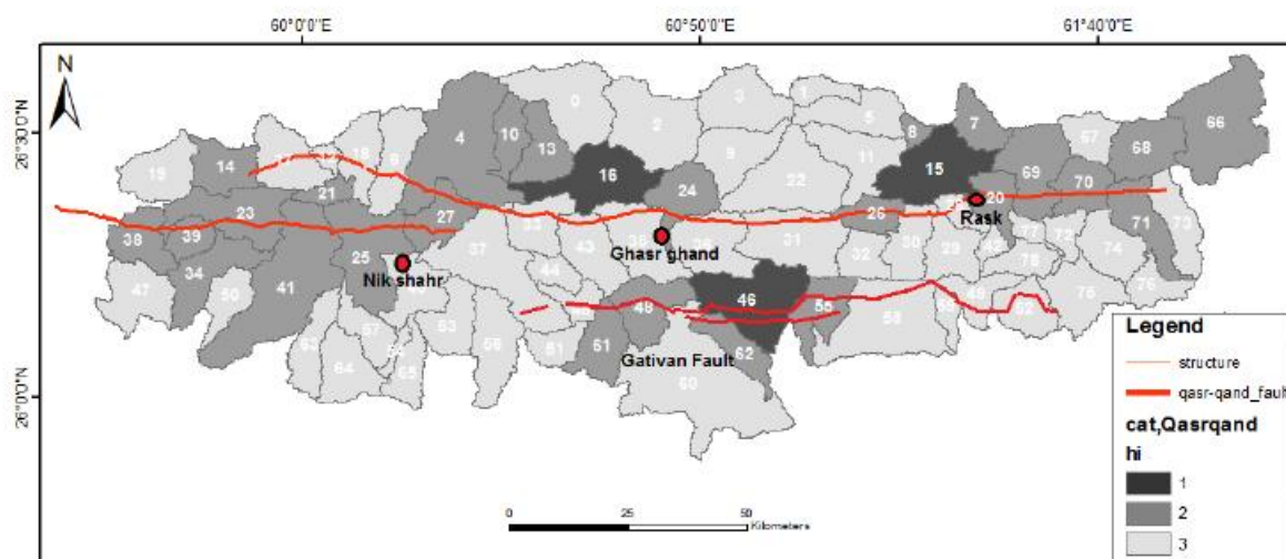
شکل ۶. نقشهٔ فزاینده‌سنجی روی حوضه‌ها و آبراهه‌های در ارتباط با راندگی‌های قصرقند، کهورکان و گتیوان. شماره‌های درج شده در نقشه نمایانگر شمارهٔ زیرحوضه‌هاست.
