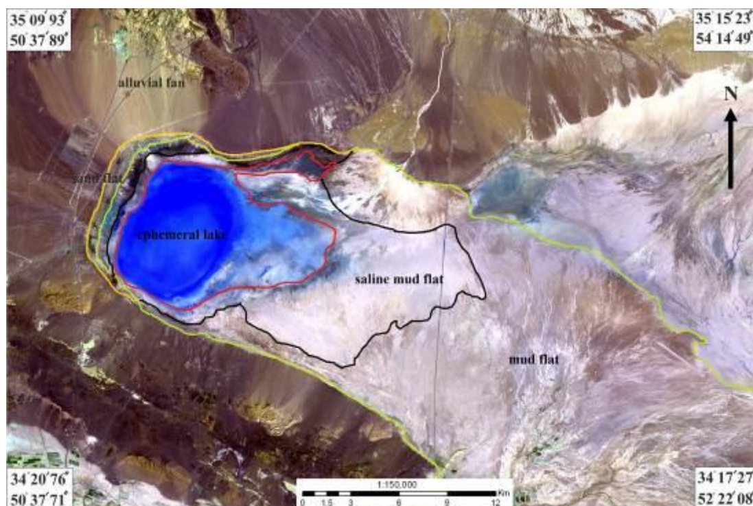
شکل ۶. الف) تفکیک زیرمحیط‌های رسوبی پلایای حوض سلطان (تصویر مربوط به دوره آبرفتی) (LANDSAT, 2004)
