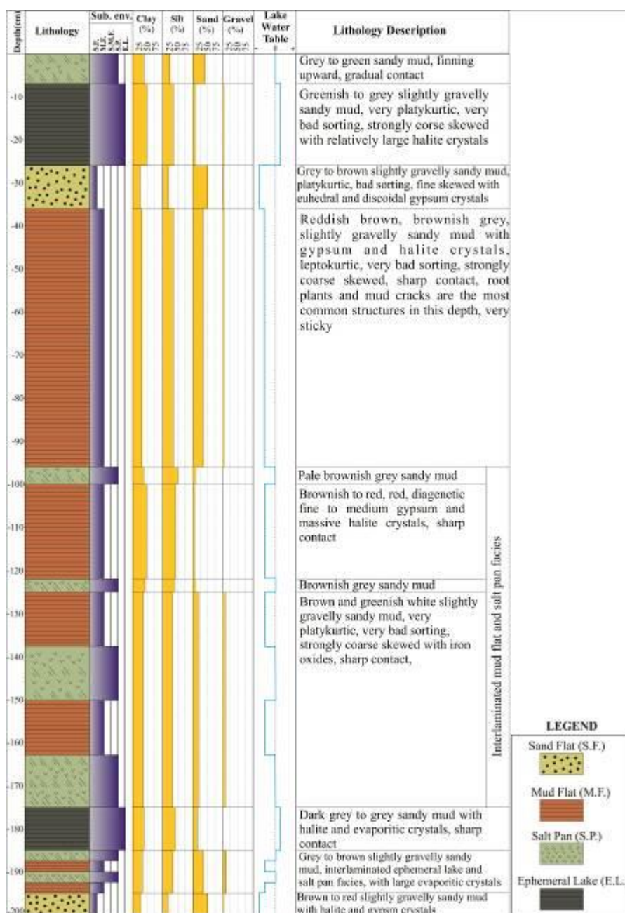
شکل ۷. ستون چینه‌شناسی، زیرمحیط رسوبی، دانه‌بندی، نوسان تراز آب دریاچه و توصیف کلی مغزه HS4
