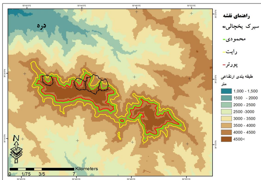
شکل ۷. برف‌مرز دائمی به روش‌های پורתر، رایت و پیشنهادشده محمودی (۱۳۶۷) در کوه شاه‌البرز
