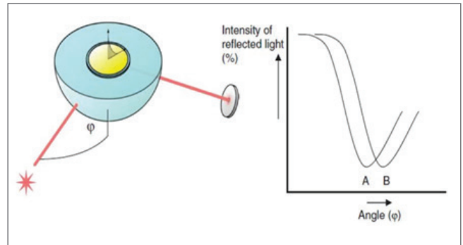
شکل ۱ شماتیک چیدمان آزمایشگاهی تحریک پلاسمون رزونانسی سطح. یک تراشه سنسور با پوشش طلا روی نیم‌کره (یا منشور) قرار می‌گیرد. نور پلاریزه از منبع نور (ستاره) به سنسور تابش می‌شود. شدت نور بازتابشی در اشارساز اندازه‌گیری می‌شود. در یک زاویه معین تابش (AE)، تحریک پلاسمون سطح اتفاق می‌افتد که نتیجه آن کاهش شدت نور بازتابشی است (A). تغییر در ضریب شکست در سطح فیلم طلا موجب جابه‌جایی زاویه از A به B می‌شود.
