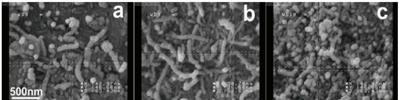
شکل ۲ تصویر SEM نانوکامپوزیت کربن چنددیواره با درصدهای a: ۵ درصد، b: ۱۰ درصد و c: ۲۰ درصد درون بستر نانوذرات تیتانیای آلاییده به نانوذرات نقره
