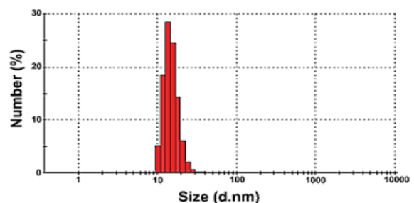
شکل ۳ توزیع اندازه ذرات کلئید نقره سیتراتی
