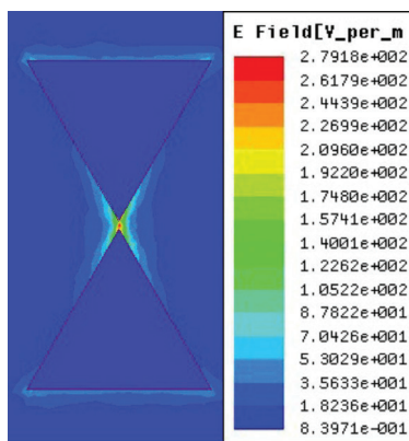
شکل ۳ توزیع میدان الکتریکی آنتن پایپونی در فرکانس تشدید
