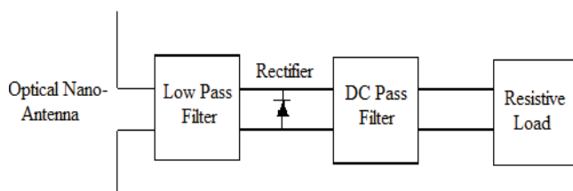
شکل ۱ | بلوک دیاگرام سیستم رکتانا دارای بار مقاومتی
