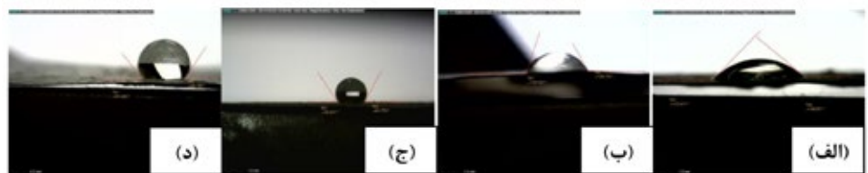
شکل ۴ زاویه تماس سطح الیاف. (الف) PVA (ب) PVA-Ag (ج) PCL (د) PCL-Ag
