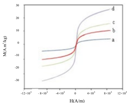
شکل ۱۰ ◀◀ حلقه پسماند نانوذرات فریت منیزیم در دماهای ۶۷۳ (a)، ۷۷۳ (b)، ۷۷۳ (c)، ۸۷۳ (d) ۹۷۳
