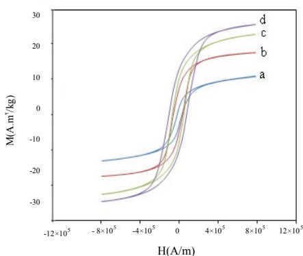
شکل ۱۱ ◀◀ حلقه پسماند نانوذرات فریت مس در دماهای ۶۷۳ (a)، ۷۷۳ (b)، ۷۷۳ (c)، ۸۲۳ (d)
