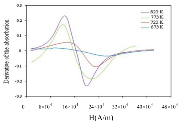
شکل ۱۴ | طیف EPR برای نانوذرات فریت مس
