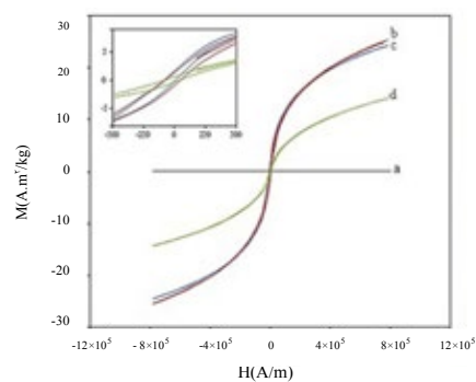
شکل ۱۲ ◀◀ حلقه پسماند نانوذرات فریت کادمیم در دماهای (a) درغیاب دمای کلسینه (b) ۶۷۳ (c)، ۷۷۳ (d) ۷۷۳
