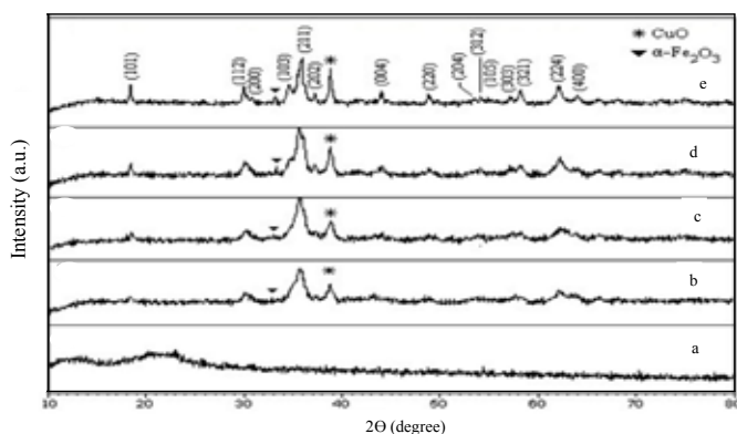
شکل ۲ پراش پرتو ایکس برای نانوذرات فریت مس در دماهای (a) درغیاب دمای کلسینه، (b) 673 ، (c) 723 ، (d) 773 ، (e) 823
