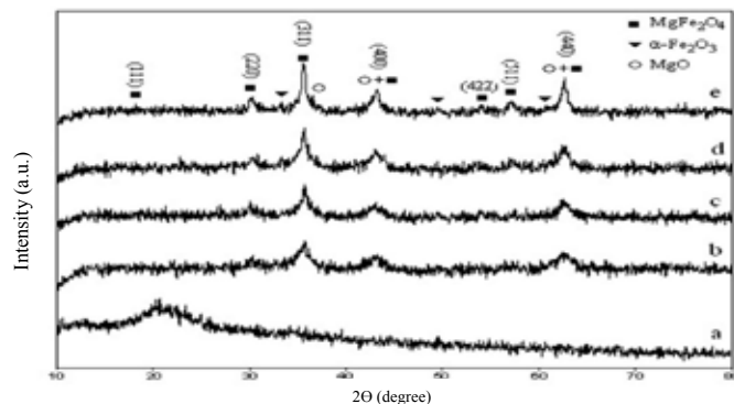
شکل ۱ پراش پرتو ایکس برای نانوذرات فریت منیزیم در دماهای (a) درغیاب دمای کلسینه، (b) 673 ، (c) 773 ، (d) 873 ، (e) 973
