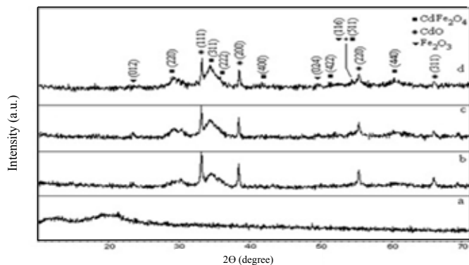
شکل ۳ پراش پرتو ایکس برای نانوذرات فریت کادمیم (a) در غیاب دمای کلسینه، (b) 673 ، (c) 723 ، (d) 773
