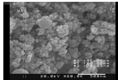
شکل ۳ تصاویر SEM نانوذرات هسته-پوسته Fe_3O_4@SiO_2 با طول مقیاس الف ( 2 \mu m ، ب ( 1 \mu m ، ج) 500 \text{ nm} .
