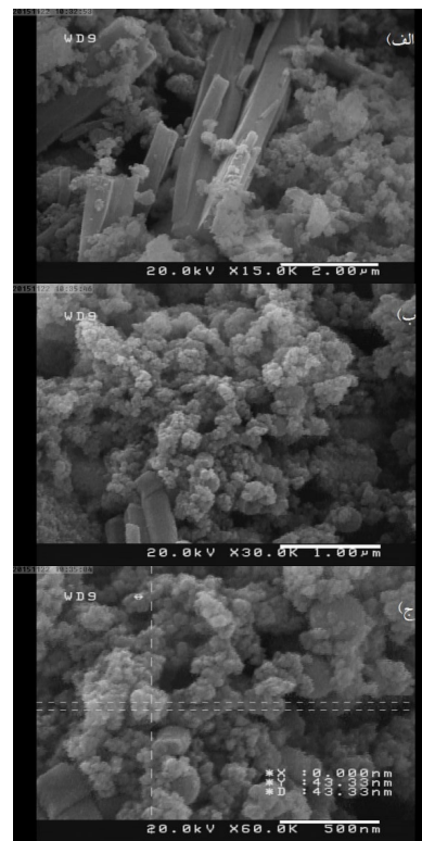
شکل ۴ تصاویر SEM مغناطیسی امید دار شده با طول مقیاس الف ( 2 \mu m ، ب ( 1 \mu m ، ج) 500 \text{ nm} .
