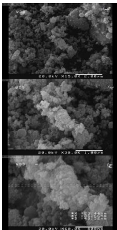
شکل ۲-۲ تصاویر SEM نانوذرات هسته-پوسته \text{Fe}_3\text{O}_4\text{-SiO}_2 با طول مقیاس الف) ۲ \mu\text{m} ، ب) ۱ \mu\text{m} ، ج) ۵۰۰nm.
