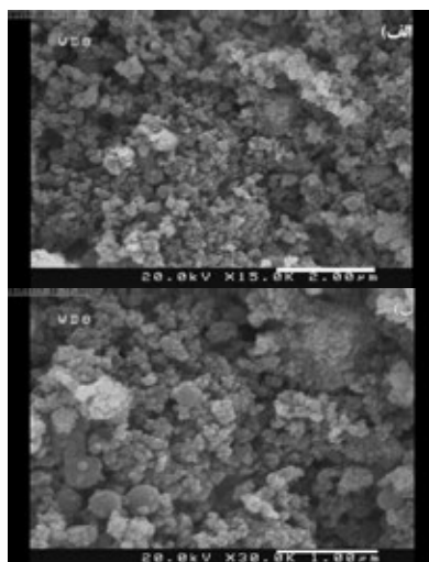
شکل ۲-۲ تصاویر SEM نانوذرات هسته-پوسته \text{Fe}_3\text{O}_4\text{-SiO}_2 با طول مقیاس الف) ۲ \mu\text{m} ، ب) ۱ \mu\text{m} ، ج) ۵۰۰nm.
