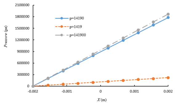
شکل ۱۴- نمودار فشار برای ۱۴۱۹، ۱۴۱۹۰ و ۱۴۱۹۰۰ ذره در جهت X
