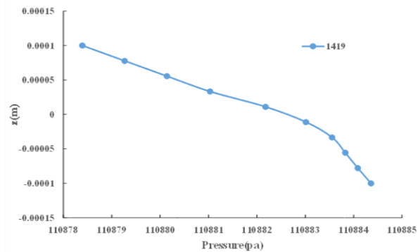
شکل ۱۱- نمودار فشار برای ۱۴۱۹ ذره در جهت Z
