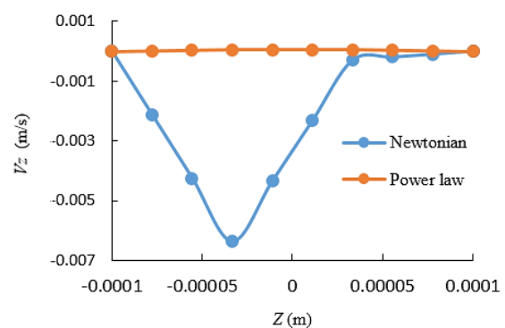
شکل ۱۰- سرعت V_z در مرکز کانال در جهت Z در دو حالت غیرنیوتنی و نیوتنی
