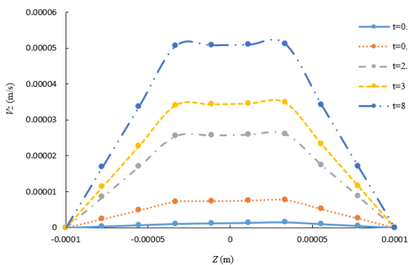
شکل ۱۳- سرعت V_z در مرکز کانال در گام‌های زمانی مختلف در جهت Z
