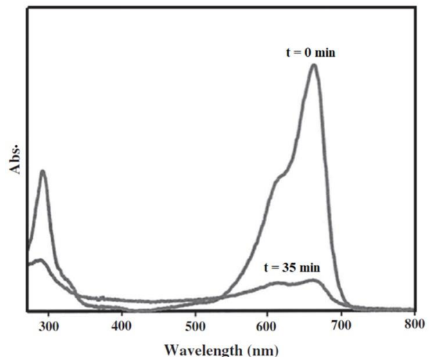
شکل ۵: تغییرات طیف جذبی رنگدانه متیلن بلو در طی فرایند فتوکاتالیستی در حضور 0/25 \text{ g L}^{-1} از نانوذرات \text{CuS} در غلظت 1/6 \text{ ppm} از رنگدانه در \text{pH}=8 .
