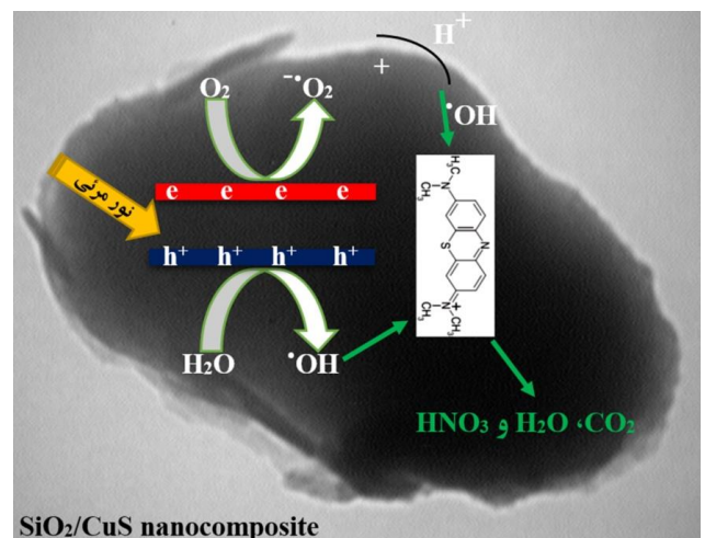
شکل ۷: مسیر محتمل برای تخریب رنگدانه متیلن بلو.
