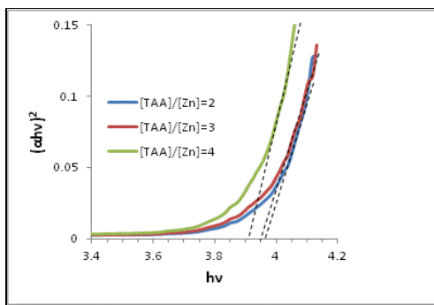
شکل ۹: تغییرات (\alpha hv)^2 بر حسب h\nu لایه‌های ZnS تهیه شده در مدت زمان ۴ ساعت لایه‌نشانی با غلظت‌های متفاوت [TAA]/[Zn]
