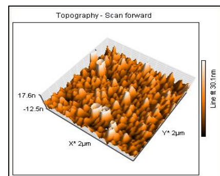
شکل ۶: تصویر AFM از لایه‌های نازک ZnS تشکیل شده بر روی زیر لایه‌ی شیشه‌ای در نسبت مولی [TAA]/[Zn 2+ ]=2 در مدت زمان ۴ ساعت لایه‌نشانی
