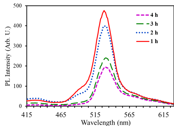
شکل ۱۰: طیف نشر فوتولومینسانس لایه‌های نازک Co: CdZnS تهیه شده در مدت زمان‌های متفاوت لایه نشانی (پیش از تزریق پیش‌ماده‌ی Zn-EDTA). دیگر پارامترها به ترتیب ۲ میلی مول از پیش ماده کبالت، ۱ میلی مول از EDTA، دمای ۸۰ °C و مدت زمان لایه نشانی ۴ ساعت (پس از تزریق پیش‌ماده‌ی Zn-EDTA) انتخاب شد.
