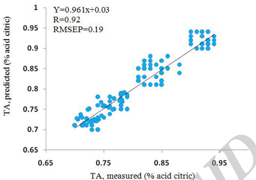
شکل (۶) مقادیر میزان pH پیش‌بینی شده توسط بهترین مدل PLS در برابر مقادیر واقعی
