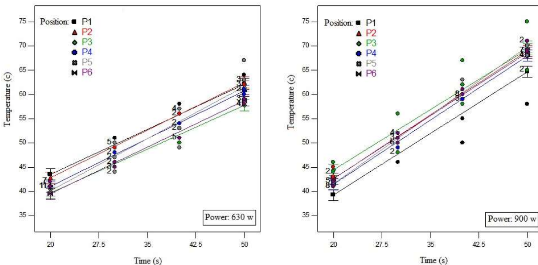
شکل (۵) نمودار اثر زمان حرارت‌دهی بر دمای محصول برای ظرف مکعبی در توان حداقل (۶۳۰w) و توان حداکثر (۹۰۰w) برای شش نقطه از محصول (P 1 , P 2 , ..., P 6 )
