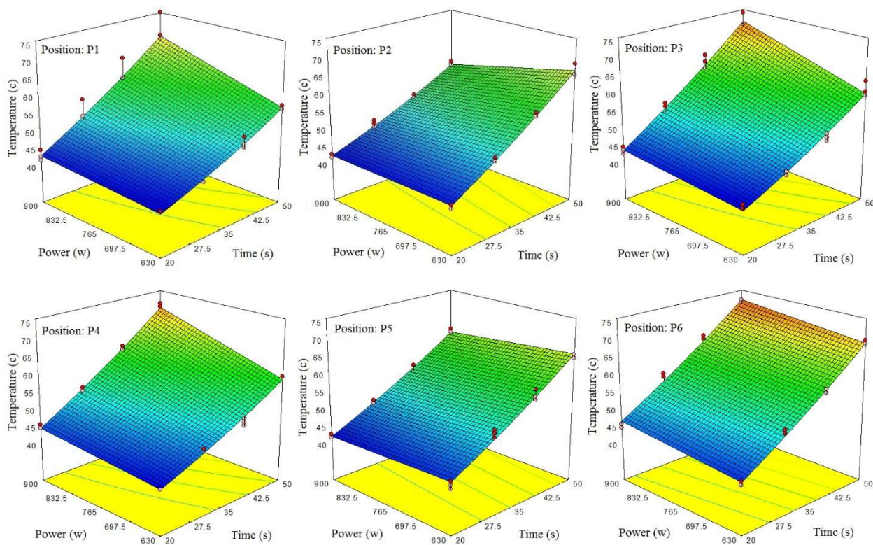
شکل (۸) نمودار سطحی اثر متقابل زمان حرارت‌دهی و توان مایکروویو در موقعیت‌های مختلف دماسنج درون محصول (ظرف استوانه‌ای)
