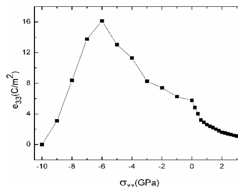
شکل ۴. تغییرات ضریب کرنش پیزوالکتریک (بالا) و ضریب تنش پیزوالکتریک (پایین) بر حسب تنش تک‌محور
