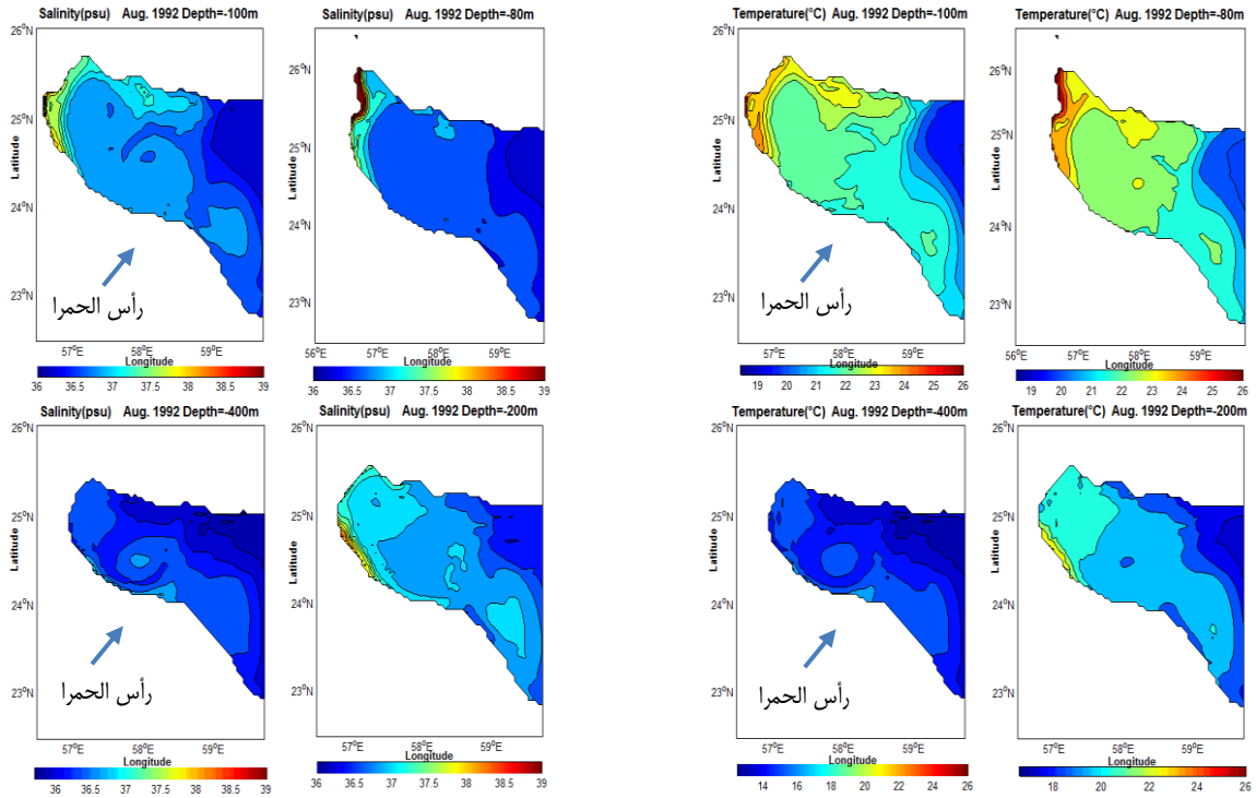
شکل ۷. میانگین ماهانه میدان شوری در عمق‌های ۴۰۰-۲۰۰-۱۰۰-۸۰ متر در آگوست ۱۹۹۲
