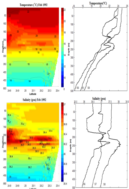
شکل ۱۱. برش های مقطعی و پروفایل قائم دما و شوری در امتداد مسیر G در شکل (۲) در زمستان ۱۹۹۲
