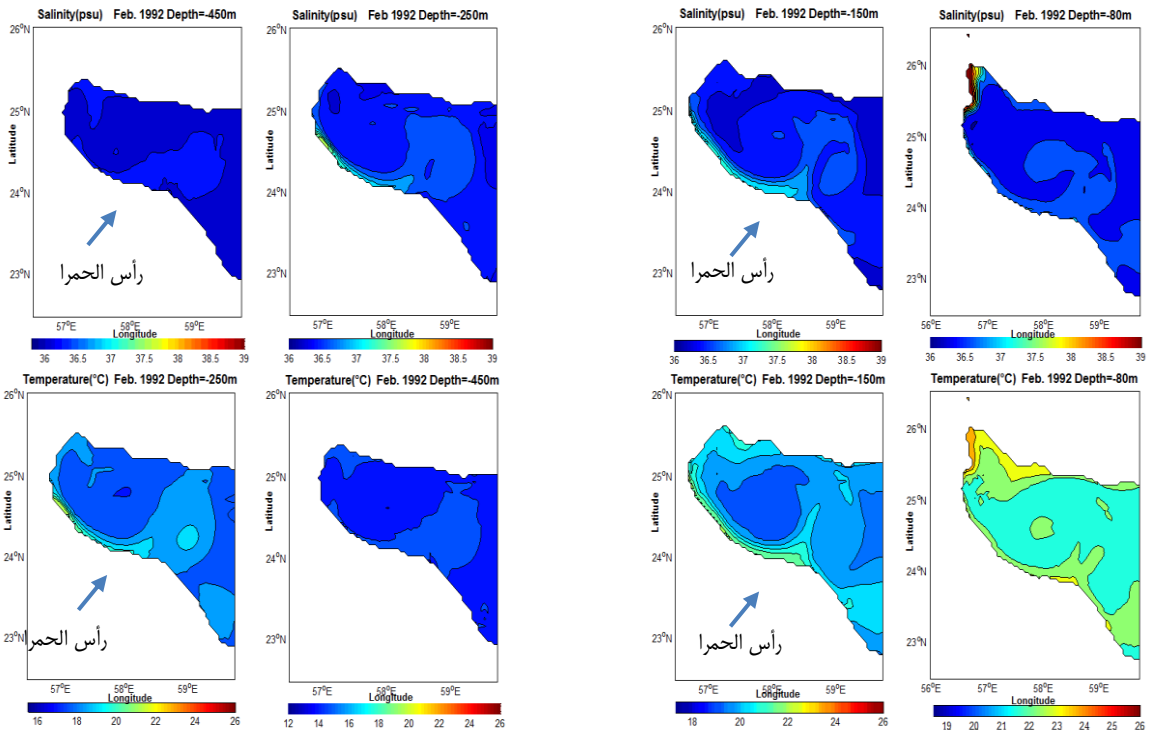
شکل ۸. میانگین ماهانه میدان شوری در عمق‌های ۴۵۰-۲۰۰-۱۵۰-۸۰ متر در فوریه ۱۹۹۲
