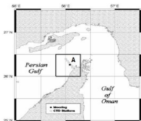
شکل ۱۳. شماتیکی از جریان ورودی و خروجی خلیج فارس در قسمت جنوبی تنگه هرمز
