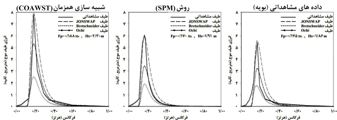
شکل ۹. طیف فرکانسی امواج برای داده های مشاهداتی (راست)، روش SPM (وسط) و شبیه سازی هم زمان جو و موج به وسیله COAWST (چپ) برای بازه زمانی رخداد باد شمال زمستانی - ۸ تا ۱۱ ژانویه ۲۰۱۵
