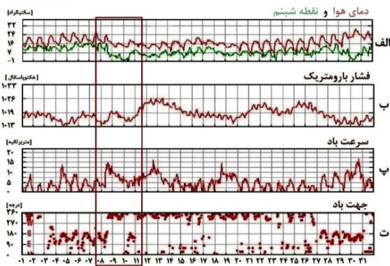
شکل ۲. نمودار الف) دمای هوا و نقطه شبینم، ب) فشار بارومتریک، پ) سرعت باد و ت) جهت وزش باد در ژانویه ۲۰۱۵ [۲۵] (کادر قرمز رنگ بازه وزش باد شمال زمستانی را نشان می‌دهد)
