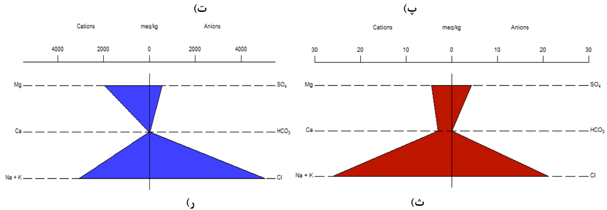
شکل ۵. دیاگرام‌های استیف برای داده‌های مربوط دشت عجب شیر و دریاچه ارومیه: الف) ریولیتی، ب) شیل، پ) آهک، ت) ژیبس، ث) آب شور، ر) دریاچه ارومیه
