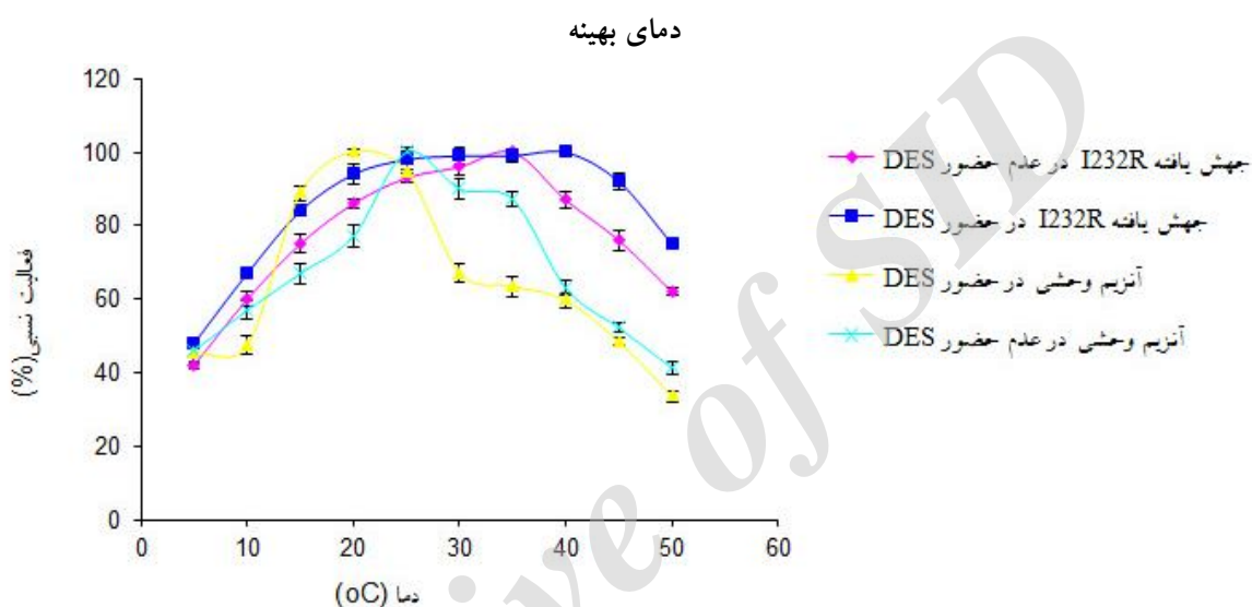
شکل 3 دمای بهینه آنزیم‌های وحشی و جهش یافته E^{354}R/Arg^{356} - I^{232}R در حضور و عدم حضور حلال DES. آنزیم جهش یافته I^{232}R - E^{354}R/Arg^{356} در شکل به اختصار I^{232}R نوشته شده است.
