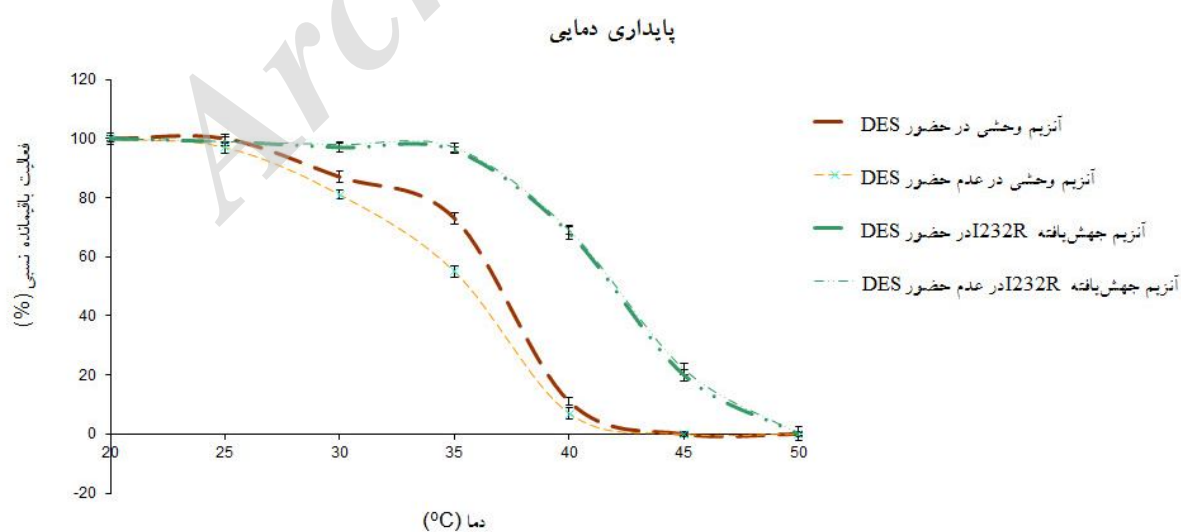
شکل 4 پایداری دمایی آنزیم‌های وحشی و جهش یافته E^{354}R/Arg^{356} - I^{232}R در حضور و عدم حضور حلال DES. آنزیم جهش یافته E^{354}R/Arg^{356} - I^{232}R در شکل به اختصار I^{232}R نوشته شده است.
