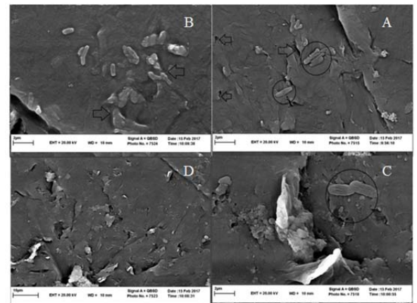
شکل ۳) تصاویر به‌دست‌آمده توسط میکروسکوپ الکترونی از سطح TLDPE پس از تاثیر گونه IRN11 در مدت سه ماه گرمخانه‌گذاری؛ (A) تکثیر باکتری روی سطح و ایجاد سوراخ‌شدگی (B، ×۵۰۰۰۰)، روزنه‌های عمیق ناشی از تاثیر باکتری (C، ×۵۰۰۰۰)، تشکیل تجمعات پرسول میکروبی در بستر بیوفیلم (D، ×۲۰۰۰۰)، ادغام باکتری و پلی‌اتیلن در اثر نفوذ باکتری (×۲۰۰۰۰)
