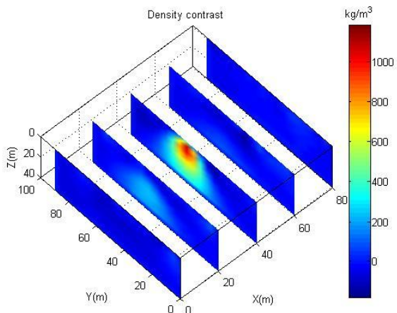
شکل ۶: نتایج وارون سازی برای مدل مکعبی در وضعیت با نوفه ۵ درصد (برش X).
