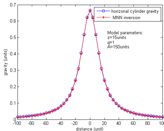
شکل ۸: میدان گرانی مدل استوانه افقی و میدان گرانی حاصل از پارامترهای مدل محاسبه شده توسط شبکه عصبی مدولار
