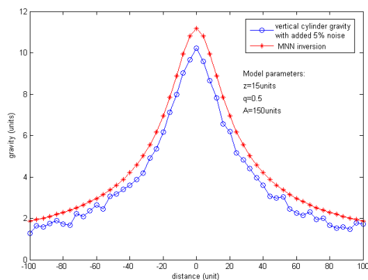
شکل ۱۰: تغییرات میدان گرانی در طول پروفیل برای مدل مصنوعی استوانه عمودی با ۵٪ نوفه تصادفی اضافه شده و میدان گرانی که از پارامترهای محاسبه شده توسط شبکه عصبی مدولار حاصل شده است
