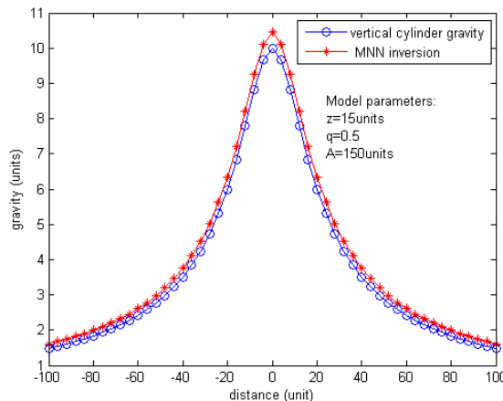
شکل ۷: میدان گرانی مدل استوانه عمودی و میدان گرانی حاصل از پارامترهای مدل محاسبه شده توسط شبکه عصبی مدولار
