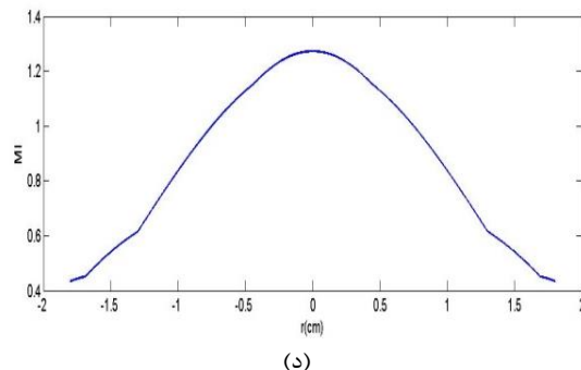
شکل ۷ (الف) منحنی تغییرات شاخص مکانیکی 0.40 . (ب) شاخص مکانیکی 0.51 (ج) شاخص مکانیکی 0.75 . (د) شاخص مکانیکی 0.89 برحسب طول محوری مسیر تابش (فاصله 0.5 سانتی‌متری از تراگذار). محور عمودی (MI) شاخص مکانیکی و محور افقی (r) راستای محور شعاعی تراگذار فراصدايي بر حسب سانتی‌متر است.
