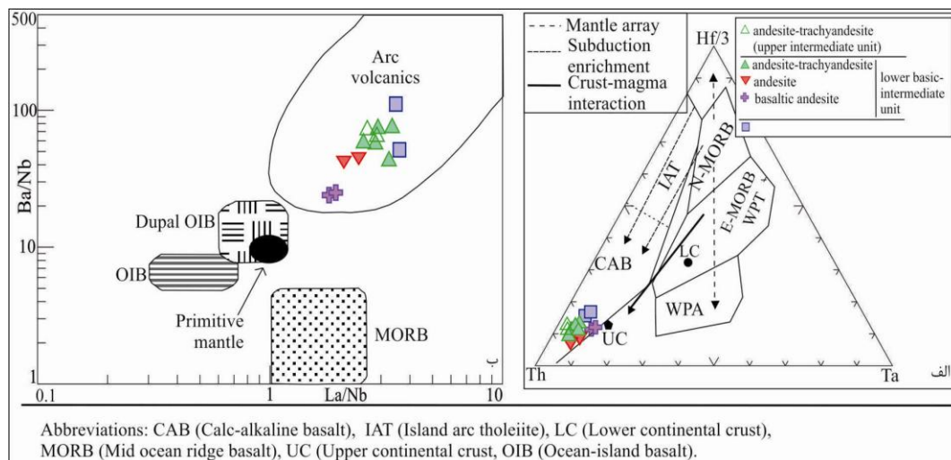
شکل ۱۰. موقعیت گدازه‌های آتشفشانی ائوسن باختر سه چنگی در نمودارهای تکتونوماگمایی، (آ) موقعیت نمونه‌های بازیک-حدواسط روی نمودار پیشنهادی [۶۶]، (ب) نمودار نسبت La/Nb به Ba/Nb به نقل از [۶۹] و سپس [۷۰]
