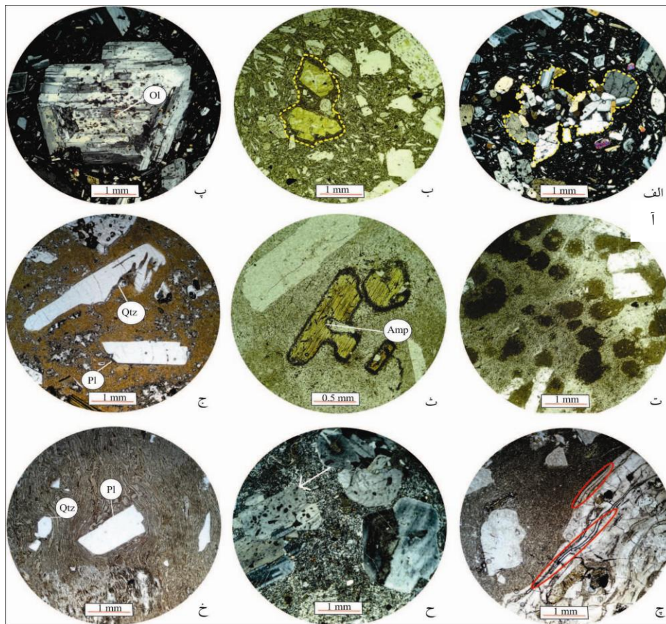
شکل ۵. (آ) انبوه‌های کومولوفیری در گدازه تراکی آندزیتی پیروکسن‌دار (XPL-4X)، (ب) میکروآنکلاوهای الیوین و پیروکسن‌دار با خمیره‌ای ریزبلور در تراکی آندزیت پیروکسن‌دار (PPL-4X)، (پ) میانبارهای الیوین در فنوکریست پلاژیوکلاز در تراکی آندزیت پیروکسن‌دار (XPL-4X)، (ت) خمیره شیشه‌ای نامتجانس در گدازه تراکی آندزیتی آمفیبول‌دار (PPL-4X)، (ث) خوردگی و انحلال در فنوکریست هورنبلاند با حاشیه اکسیده در گدازه تراکی آندزیتی آمفیبول‌دار (PPL-10X)، (ج) فنوکریست کوارتز با خوردگی‌های خلیجی در ریولیت پورفیریک (PPL-4X)، (چ) فیام‌ها و پسودوفیام‌ها را در تراکی داسیت هیبریدی نشان می‌دهد که از اطراف توسط کانی‌های ایک احاطه شده‌اند. نیمه بالایی تصویر پسودوفیام آندزیتی-تراکی آندزیتی پورفیریک است (PPL-4X)، (ح) بافت اسفنجی در فنوکریست پلاژیوکلاز در گدازه تراکی داسیت میکروکریستالین (XPL-4X). (خ) بافت اوتاکسیتی را در ریولیت واحد اسیدی زیرین نشان می‌دهد (PPL-4X).
