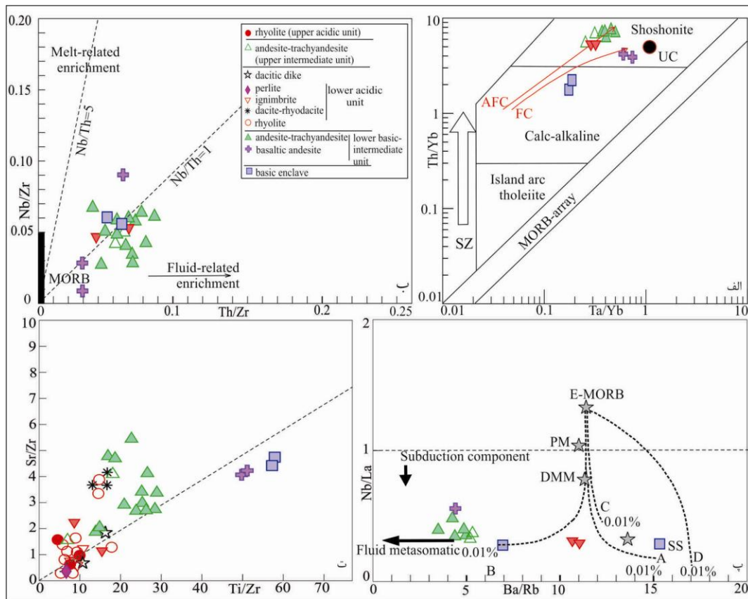
شکل ۱۱. (آ) نمودارهای ژئوشیمیایی برای تعیین منشأ سنگ‌های بررسی شده را نشان می‌دهد. (آ) از [۶۷]، (ب) از [۷۳]، (پ) از [۷۴] است. ترکیب گوشته اولیه (PM) و E-MORB از [۵۳] است و میانگین ترکیب گوشته نهی شده (DMM) و رسوبات فرورانشی (SS) به ترتیب از [۷۵] و [۷۶] است. B، C و D به ترتیب نشان‌دهنده ترکیب گارنت لرزولیت [۷۷]، گارنت-آمفیبول لرزولیت [۷۸]، گارنت-آمفیبول-فلوگوپیت لرزولیت [۷۸] و فلوگوپیت-گارنت هارزبورژیت [۷۴] هستند، (ت) از [۵۲]، که نشان‌دهنده نقش آمیختگی ماگمای حاصل از ذوب‌بخشی گوشته و ماگمای حاصل از ذوب‌بخشی پوسته‌ای در تشکیل سنگ‌های بررسی شده است.
