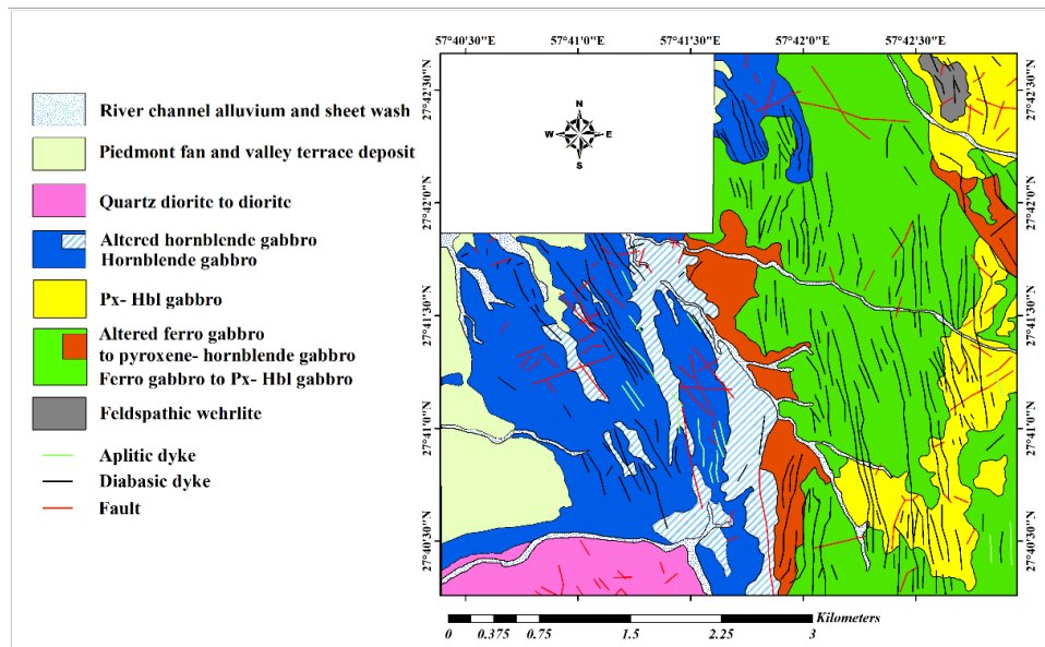
شکل ۳. نقشه زمین‌شناسی تهیه شده از آنومالی درگز با مقیاس ۱/۵۰۰۰
