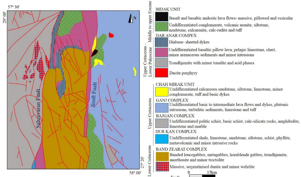
شکل ۲. نقشه زمین‌شناسی ناحیه‌ای کمپلکس افیولیتی بندزیارت-دره‌انار در مرکز که به‌وسیله گسل جیرفت از بلوک گنج و گسل سبزواران از بلوک باجگان جدا شده است ( با تغییرات از نقشه‌های زمین‌شناسی ۱/۱۰۰۰۰۰ ورقه‌های قلعه منوجان و کهنوج تهیه شده به‌وسیله زمین‌شناسان شرکت پاراگون)
