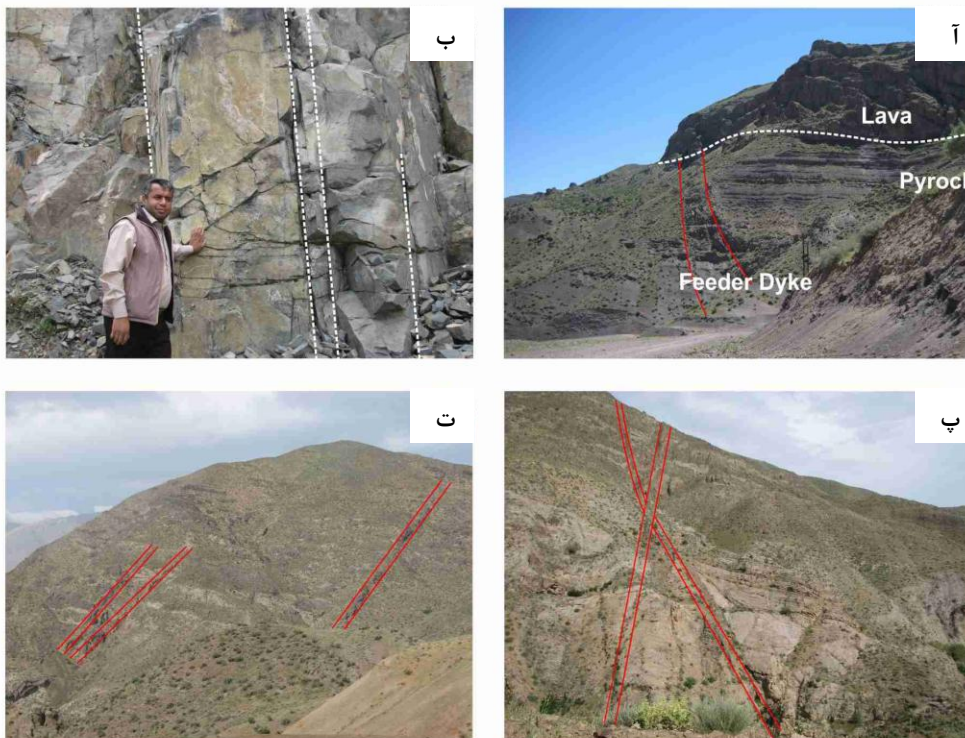
شکل ۴. روابط صحرائی رخساره‌های مختلف آتشفشانی در منطقه لات بلوکان، آ) ساختار چینه‌سان، ب) درزه‌های منشوری، پ) دایک میکرودیوریتی، ت) دایک آندزیتی
