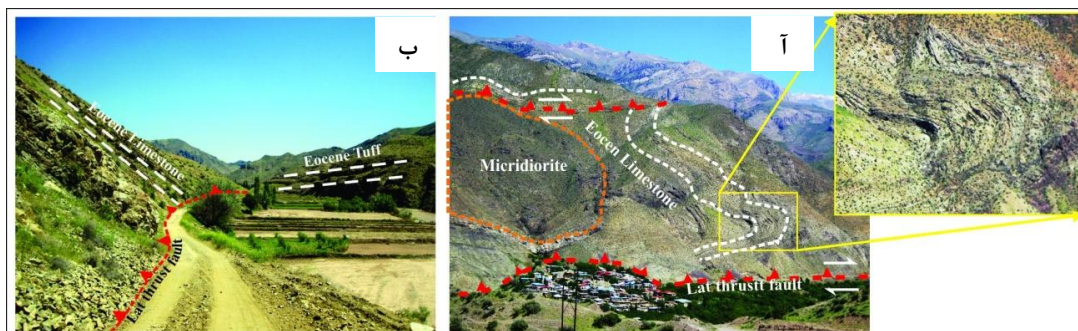
شکل ۷. آ) وجود یک چین خوابیده و روند مورب نسبت به گسل لات در شمال دره گسلی، مؤید مؤلفه لغزشی - فشارشی راست‌بر نیز هست (شمال روستای لات، دید به سمت شمال)، ب) تغییر شیب ناگهانی لایه‌بندی در دوسوی دره گسلی، شاهد گسلی بودن رودخانه شاهرود است (غرب روستای لات، دید به سمت شرق)
