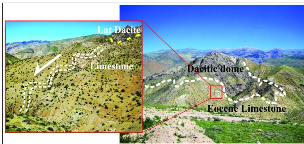
شکل ۶. گنبد داسیتی لات که در لایه‌های توفی و سنگ آهک توفی رخساره رسوبی-آذرآواری تزریق شده و موجب ایجاد چین‌های لغزشی در این لایه‌ها شده است.
