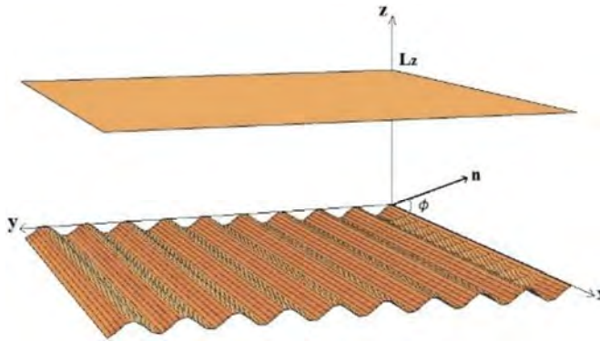
شکل ۲ هندسه مسئله تیغه بلور مایع نماتیک؛ \phi زاویه بین جهت نما و محور X (امتداد شیارها) است.
