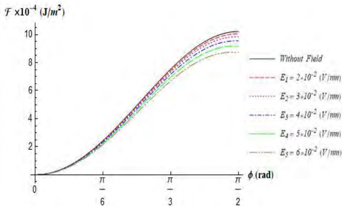
شکل ۴ تغییرات انرژی چنگ زدگی بلور مایع نematیک نسبت به زاویه \phi بدون حضور میدان الکتریکی خارجی (نمودار توپر) و در حضور میدان‌های الکتریکی با شدت‌های مختلف از 2 \times 10^{-2} V/nm تا 6 \times 10^{-2} V/nm (نمودارهای خط‌چین).
