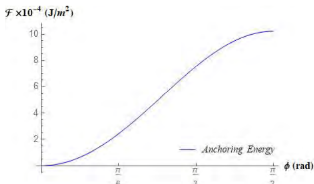
شکل ۳ انرژی چنگ‌زدگی بلور مایع نماتیک در نزدیکی سطح شیاردار در چارچوب نظریه فوکودا.
