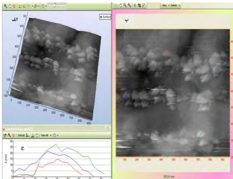
شکل ۳ تصویر (الف) تصویر سه بعدی سطح نشان دهنده ایجاد نانوساختارهای خطی با سه سرعت متفاوت (الف) از بالا به پایین ۲۰ نانومتر در ثانیه، ۴۰ نانومتر در ثانیه، ۸۰ نانومتر در ثانیه. تصویر (ب) همان سطح به صورت نمایش دوبعدی و تصویر (ج) نمودار اندازه نانوساختارهای ایجاد شده.
