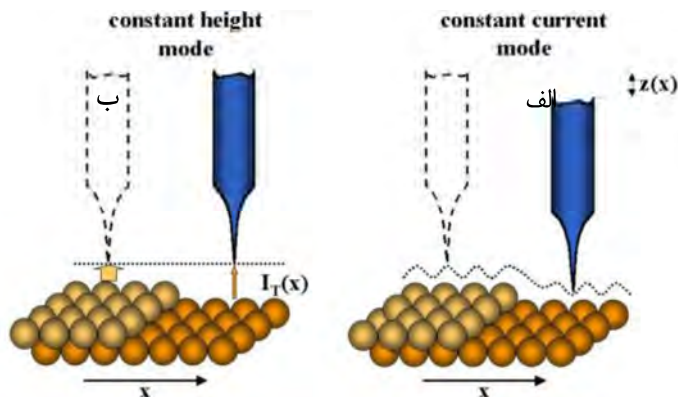
شکل ۱ مد جریان ثابت (الف) و مد ارتفاع ثابت (ب) در میکروسکوپ STM.
